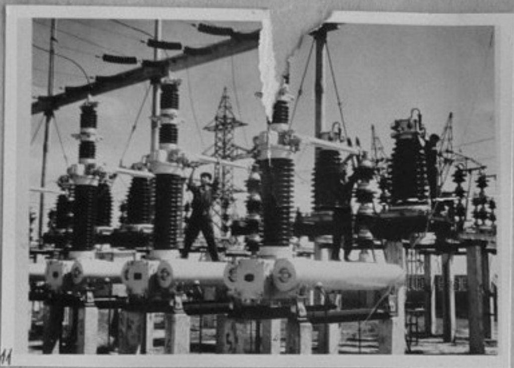
65/225-11-Електрическа станция Доинг-анх. /ММ/ 24/36
