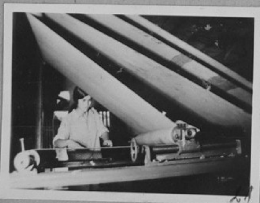
80-123-21 Хартиената фабрика "Трик Бач" - Ханой се снабди с нови две машини с годишен капацитет общо 150 тона - новите машини за производство на хартия репр./МД
