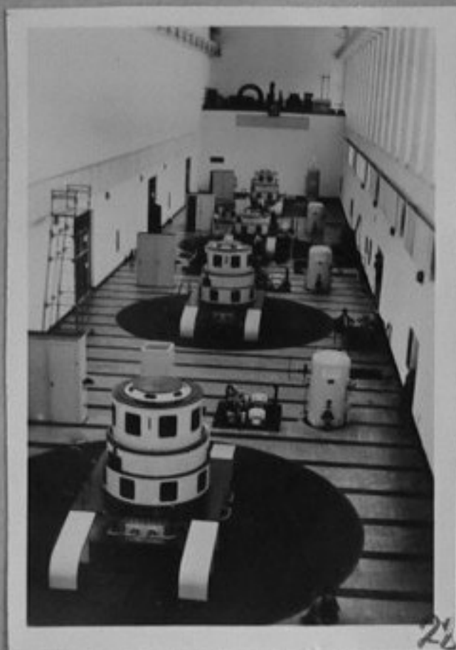
79-267-28-Изглед от турбинната зала на ВЕЦ при язовир Наглу, който събира водите на реките Кабул и Паншер в долината Наглу между Кабул и Джалалабад. /репр./ЛА
