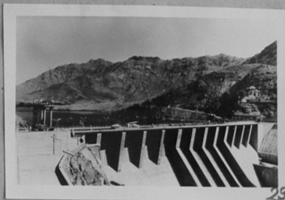
79-267-29-Язовирът "Наглу" е висок 110м. Проектът за язовир е реализиран с помощта на СССР и е внушителен пример за ефективно-то сътрудничество, което се предоставя на Афганистан от неговия съсед, за да бъде преодоляна икономическата му изостаналост. /репр./ЛА
