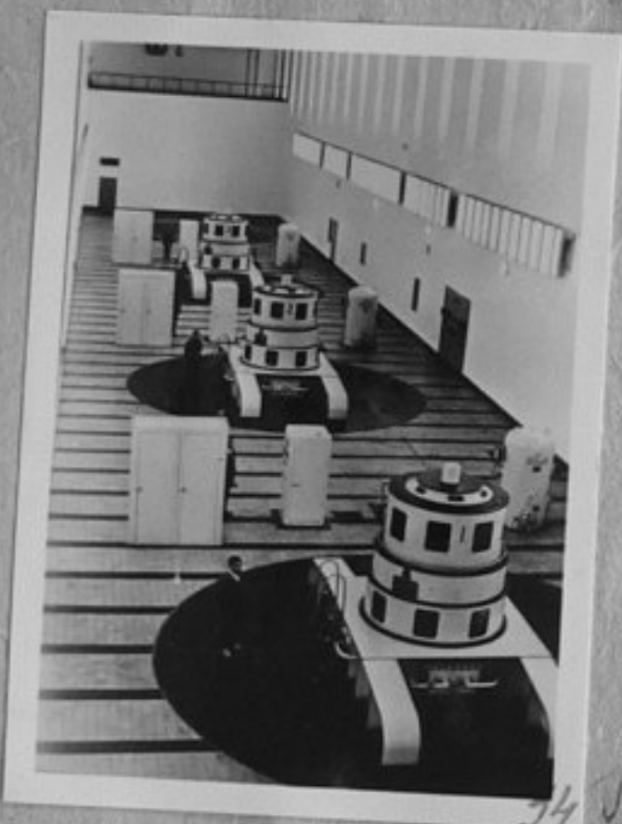
73-3227-34-Машина зала на хидроелектроцентрала в Нагла, построена при сътрудничество на СССР. /репр. П. Щерев/ТК
