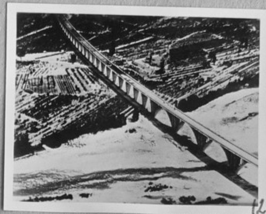
75-2585-12-Дълъг виадукт над р. Паглия по новата ж.п. линия Рим-Флоренция. /репр./ТК
