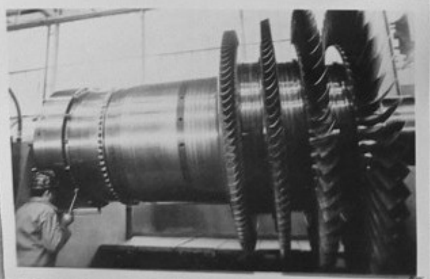
74-1580-17-Роторът на новата мощна газова турбина "Фиат ТГ 50", показан на 19-та годишна международна конференция за газови турбини в Цюрих. /Репр.П.Щерев/СС
