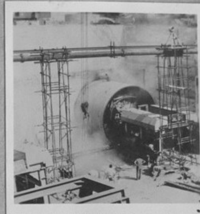
70-277-3-Строеж на новото метро в Рим. /репр./ ИК
