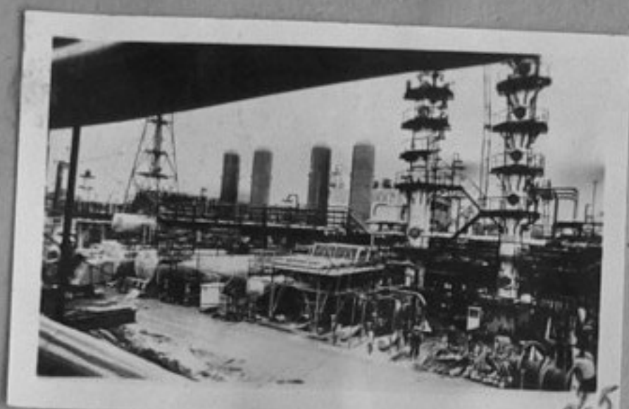
80-323-25 Ленинградская област. Комплексът за произв. на парафин "Парекс" построен към Киришския нефтепреработвателен завод. Комплексът "Парекс" ще произв. суровини за биохимич. комбинат. От парафина ще се произв. белтъч- но-витаминозен концентрат - висо- кокалорична храна за добитъка. репр./МД
