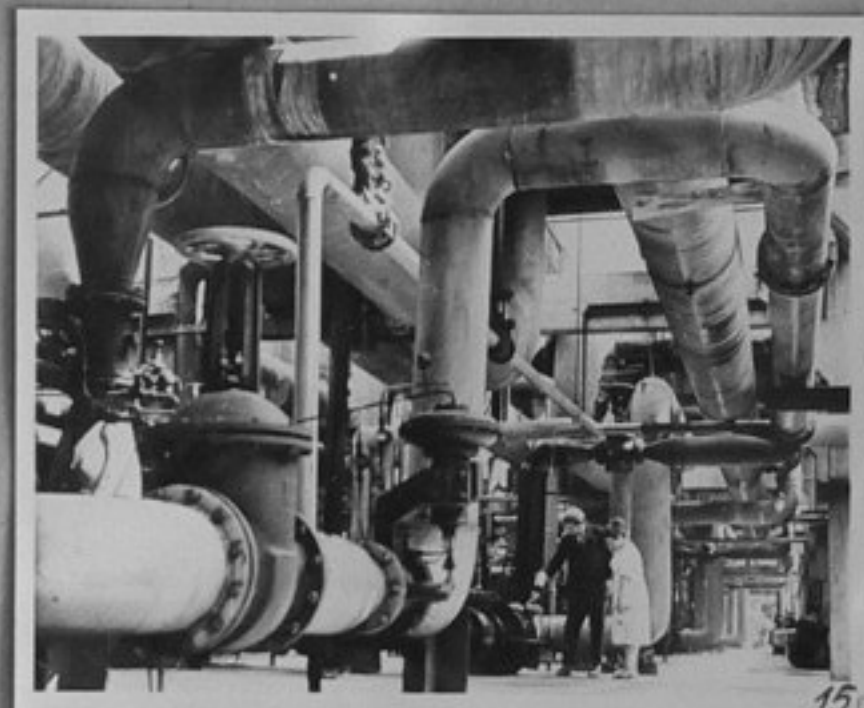
15-Изглед от цеха за конверсия на метана в Чирчикския електрохимически комбинат в Узбекистан.
