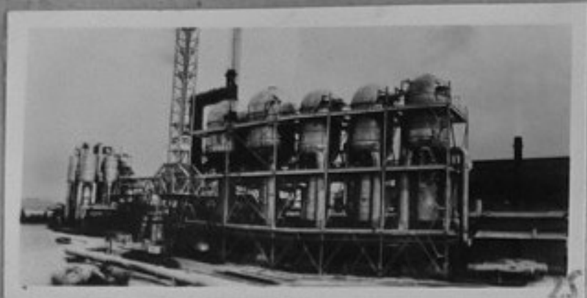
72-4342-25-Нови промишлени опреснителни съоръжения за прясна питейна вода в гр. Шевченко на полуостров Мангшлак. /репр./ ИК
