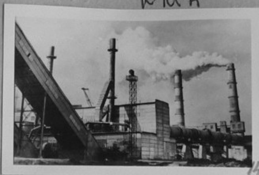
74-2179-14-Четвъртата технологична линия на Староскопския циментен завод, Белгородска област. На строежа работят български специалисти. /Репр. П.Щерев/СС
