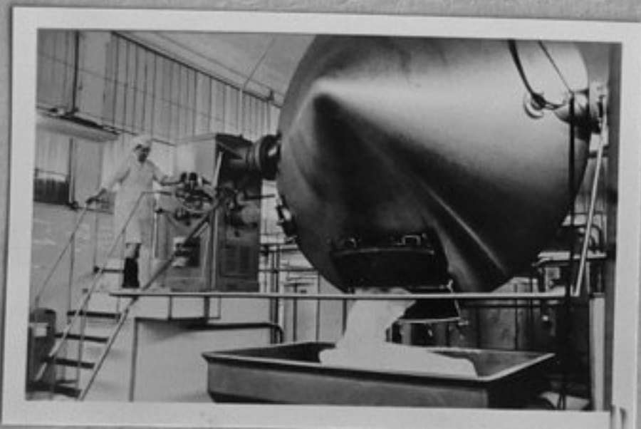
73-109-11-Изглед от цеха за масло в Млекопреработвателния комбинат във Валмиер. /Репр. П. Щерев/МК
