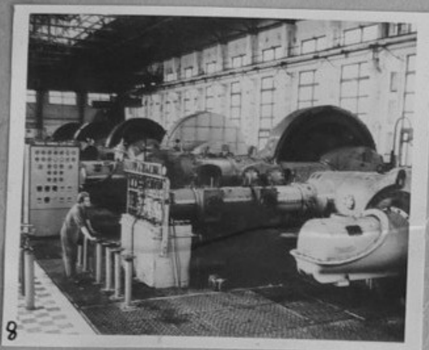
8 63/3235-8-Новият компресорен цех в Новомосковский химически комбинат, Тулска област. /ММ/
