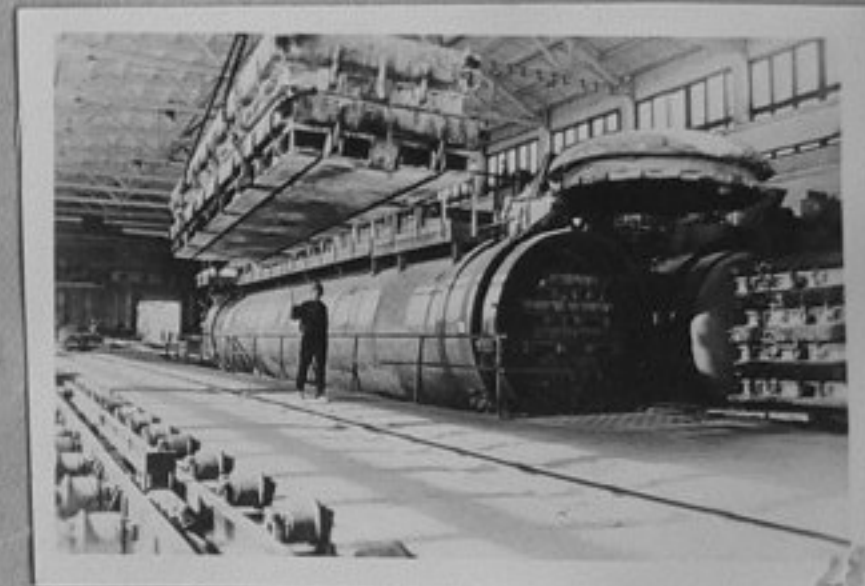
72-4250-28-Изглед от цеха за производство на аглопоритосиликатни панели в Минския комбинат за силикатни изделия. Аглопоритът е изкуствен, порест, керамичен материал. /репр./ ИК
