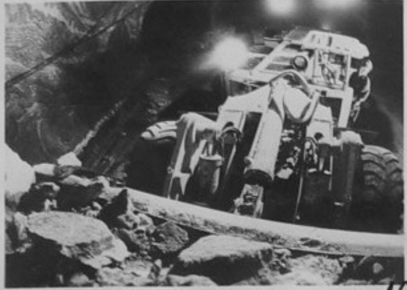
76-4057-16-Пермска област. Мощни самоходни товаро-разтоварни машини работят в забойите на втория Соликамски калиев комбинат, като осигуряват висока производителност на труда.
