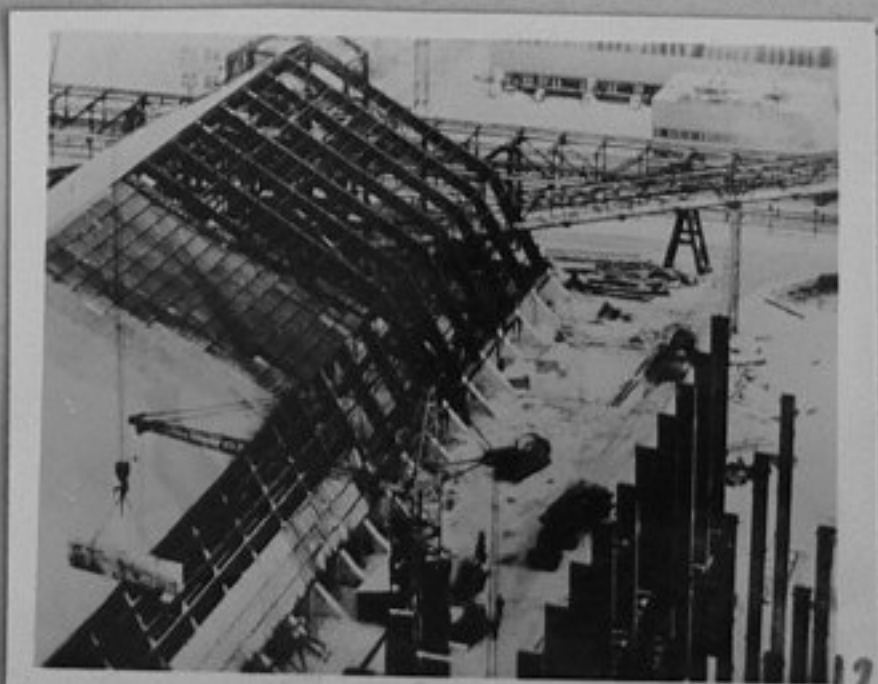
73-3862-26-Комплекс от пречиствателни съоръжения към Химическия комбинат в гр. Северодонецк, Украйна. /репр. П.Щерев/СС
