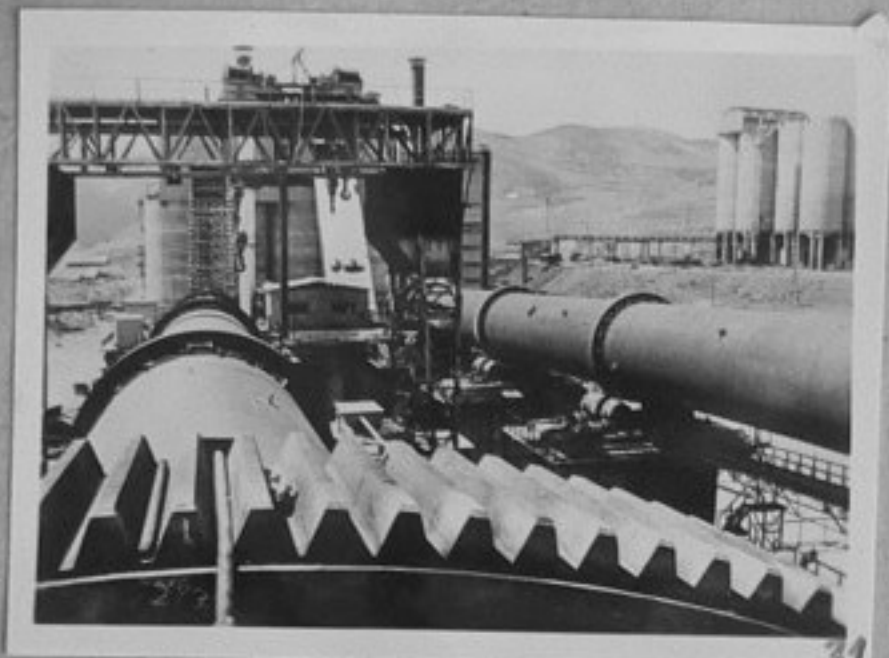
72-864-31-Общ изглед от пещта за производство на цимент в Химическия комбинат в гр.Раздан. /репр.П.Щерев/ИК
