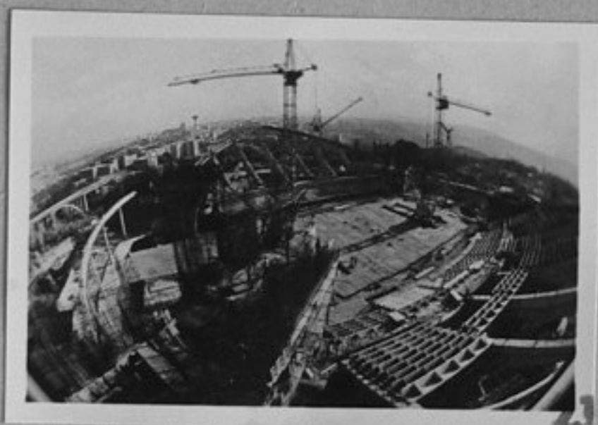
80-3819-23 В Ереван на високия хълм "Цицернакаберд" се строи един от най-големите зрелищни обекти на Армения - спортно концертният комплекс С.Метелица/МД
