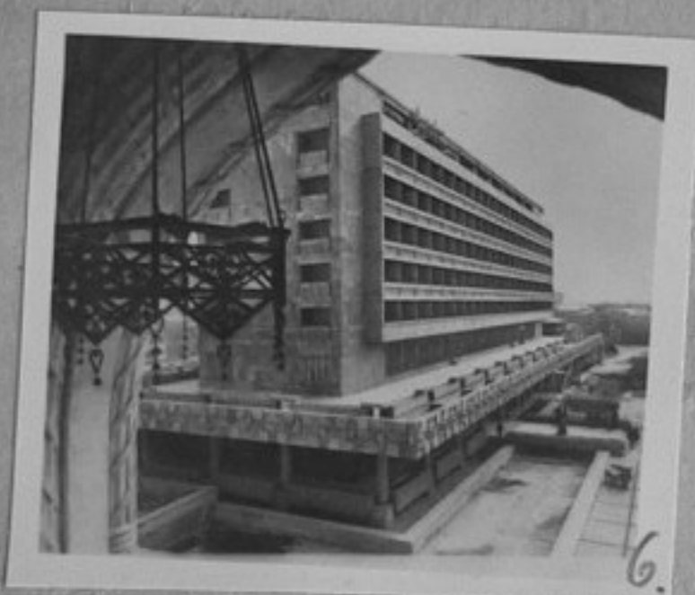
70-1759-6-Външен вид на новия хотел за 250 души "Ашхабад" в столицата на Туркмения. /репр./ ИК
