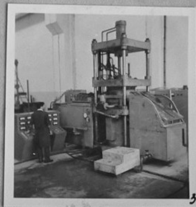
68-4012-1,2,3-Леене на метали с противовъздушно налягане по методите на проф. Балев. /Л. Чаръкчиев/ XII
