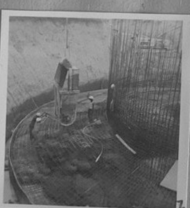
71-3636-7-Строежът на основите на 150 м. комин на АЕЦ./Л.Златков/ИК
