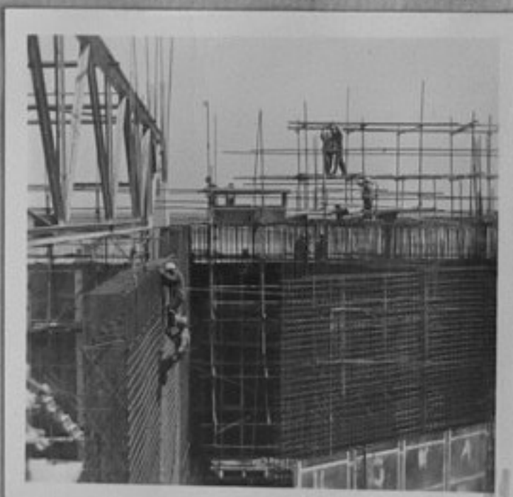
71-3589-10,11-Строежът на I АЕЦ. /Х.Сиромахов/ИК
