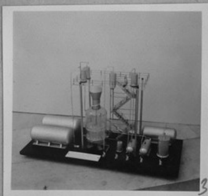
72-4841-3>Макет на техноло- гия за производство на хлорхолинхлорид с ръко- водител инж. Д. Вълчев. /Н. Чобанов/ИК
