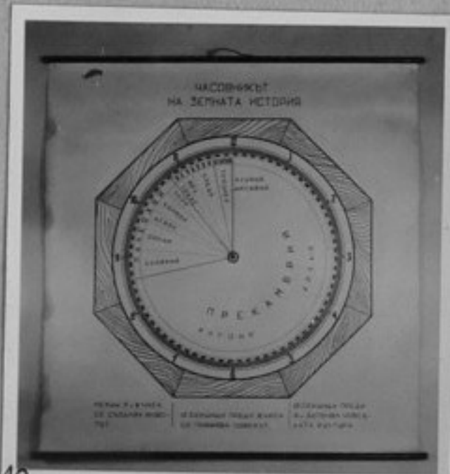
10-Часовникът на земната история.
