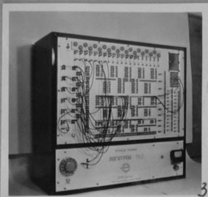
Наградени експонати от младежката изложба в гр. Пловдив, изработени от колективи при института. /Лало Златков/ ИК 71-254-Логически трена- жор "Логитрон" ТЛ-2.
