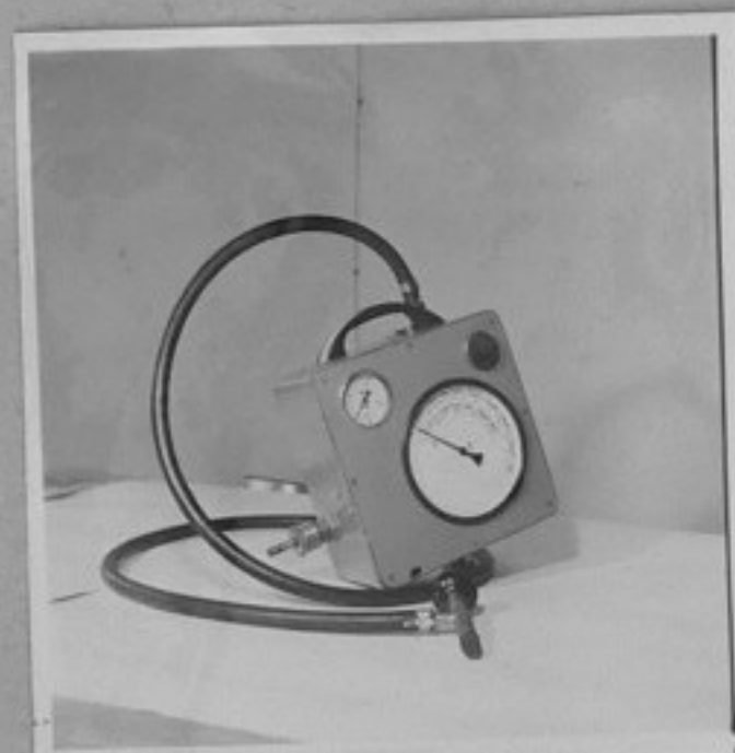
70-5799-5-Пневматичен калибратор за определяне относителната неплътност на цилиндри на двигатели с вътрешно горене. /Л.Златков/ XII
