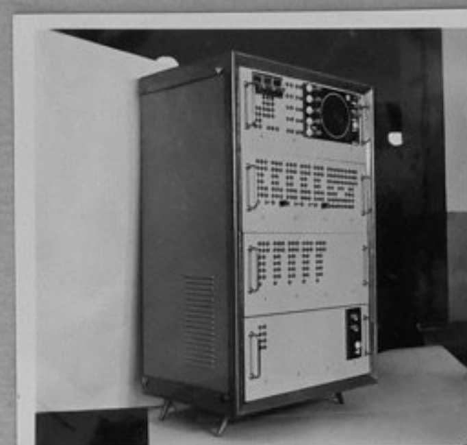
71-255-2-Устройство за електронно моделиране на топлинните процеси.
