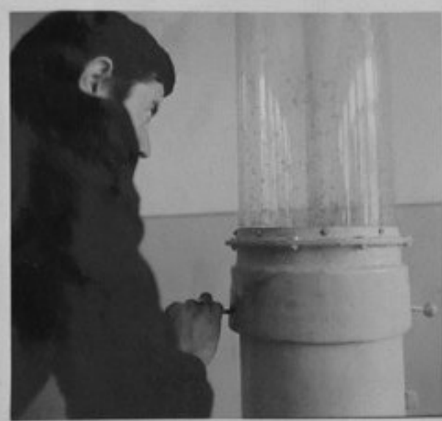
70-1694-5-Аеродинамична тръба "Класификатор" за определяне аеродинамичните свойства на зърнените материали. /Д.Рогев/ ИК
