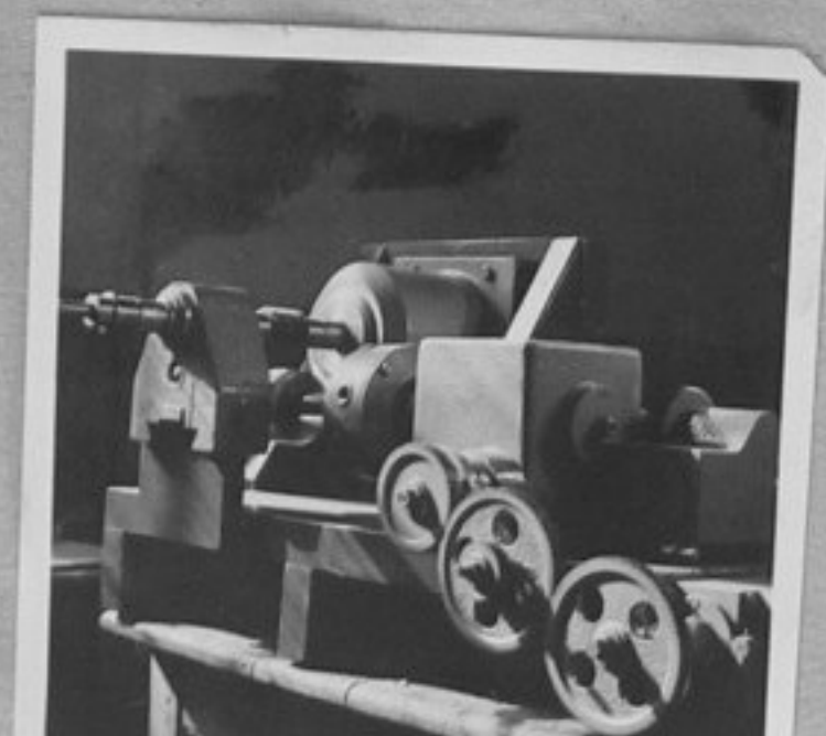
Техникум по механотехника - Габрово. 70-895-8-Приспособление за нарязване на зъбни козела с червячна модулна фреза на универсална фрезова машина.
