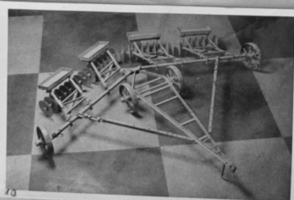
63/928-10,12 - Люцилник ЛБД-45 и култиватор КУТС-4.20 /макети/ изработени от курсистите при техникума за механиз. на селското стоп., Ямбол. /Йорданов/ ММ
