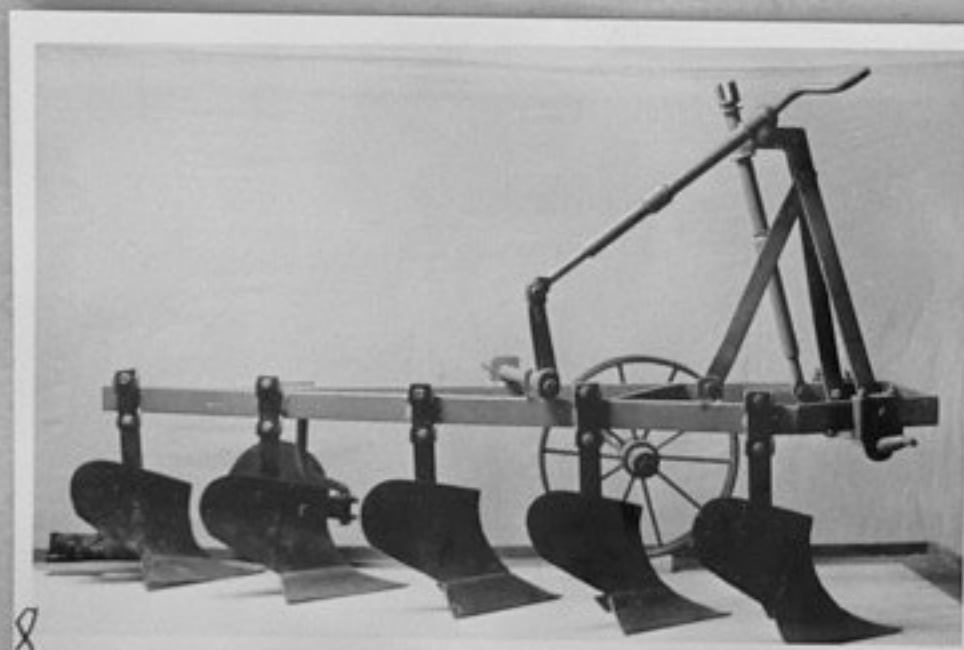
8-Техникум по механиз. на селското стоп. - навесен плуг ПН-5-30. /Ямбол/
