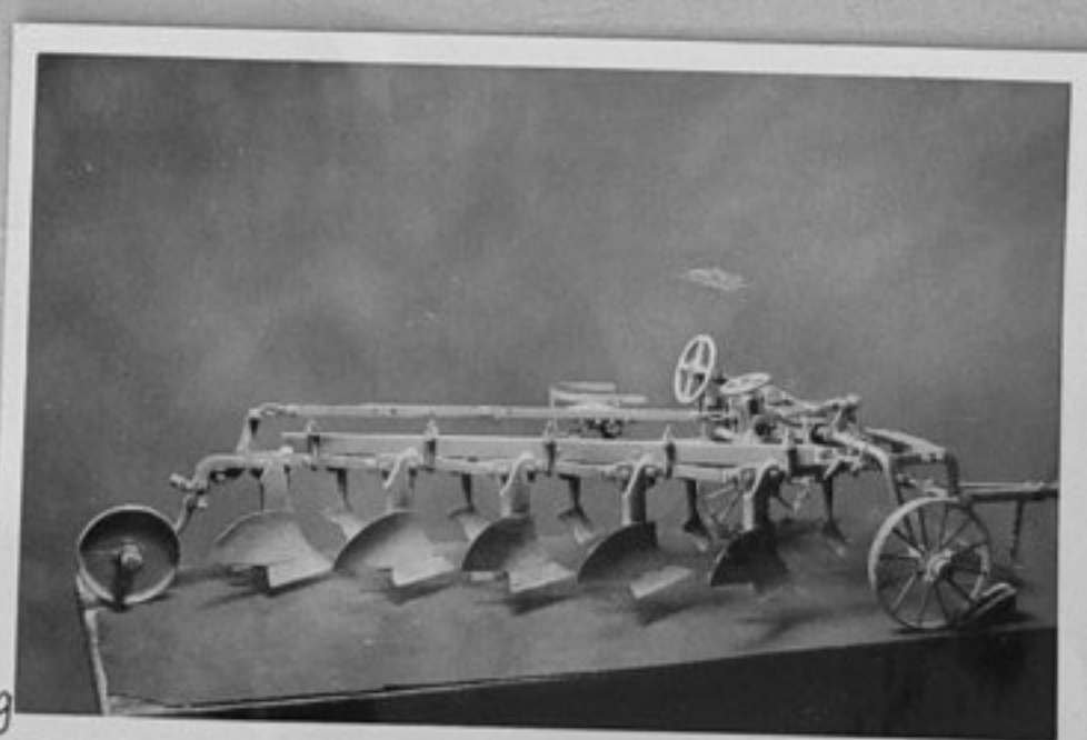
9-Техникум по механиз. на сел. стоп. - прекачен плуг П-5-30. /Ямбол/
