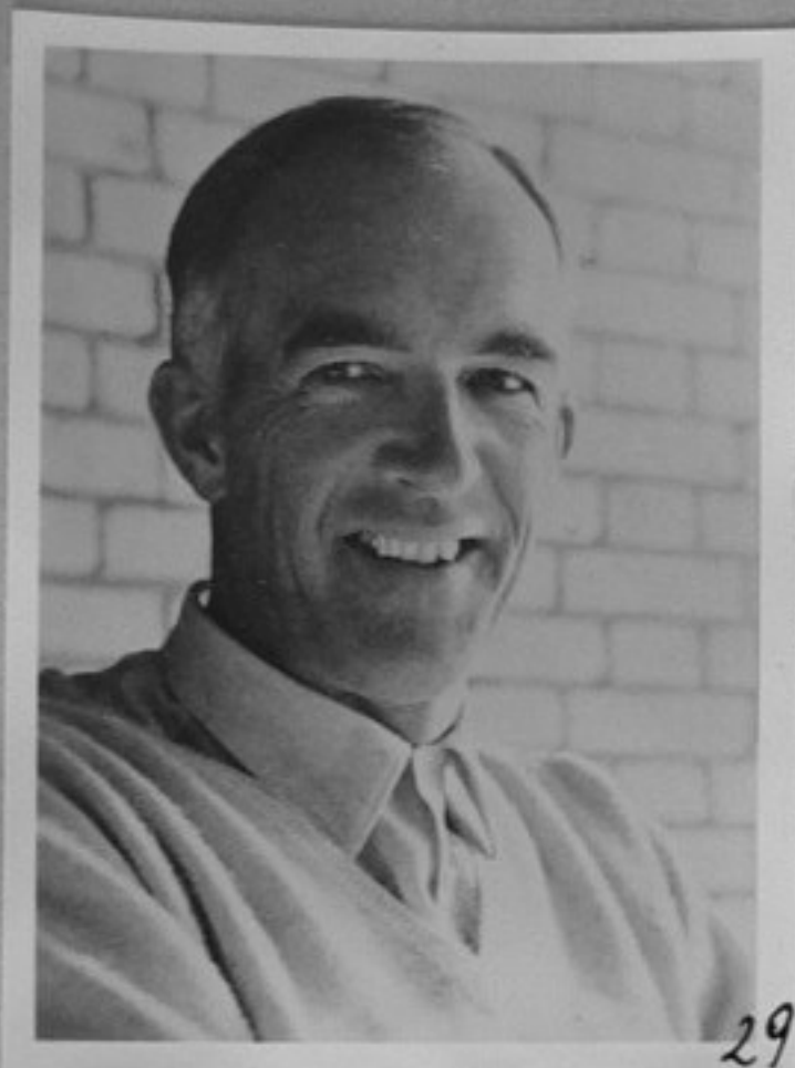
68-4848-29-Йорн Утзон, дат- ски архитект, род. 9.4.1918 в Копенхаген. /Репр./ ХП
