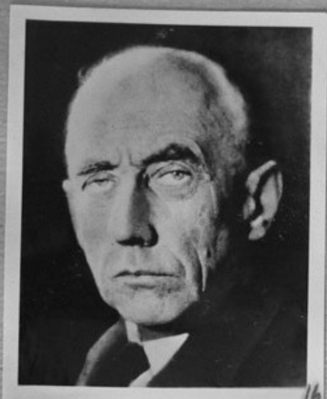
68-6153-16- Амундсен, Раул /1872-1928/ - нор- вежски полярен пъте- шественик и изследова- тел. /СС/
