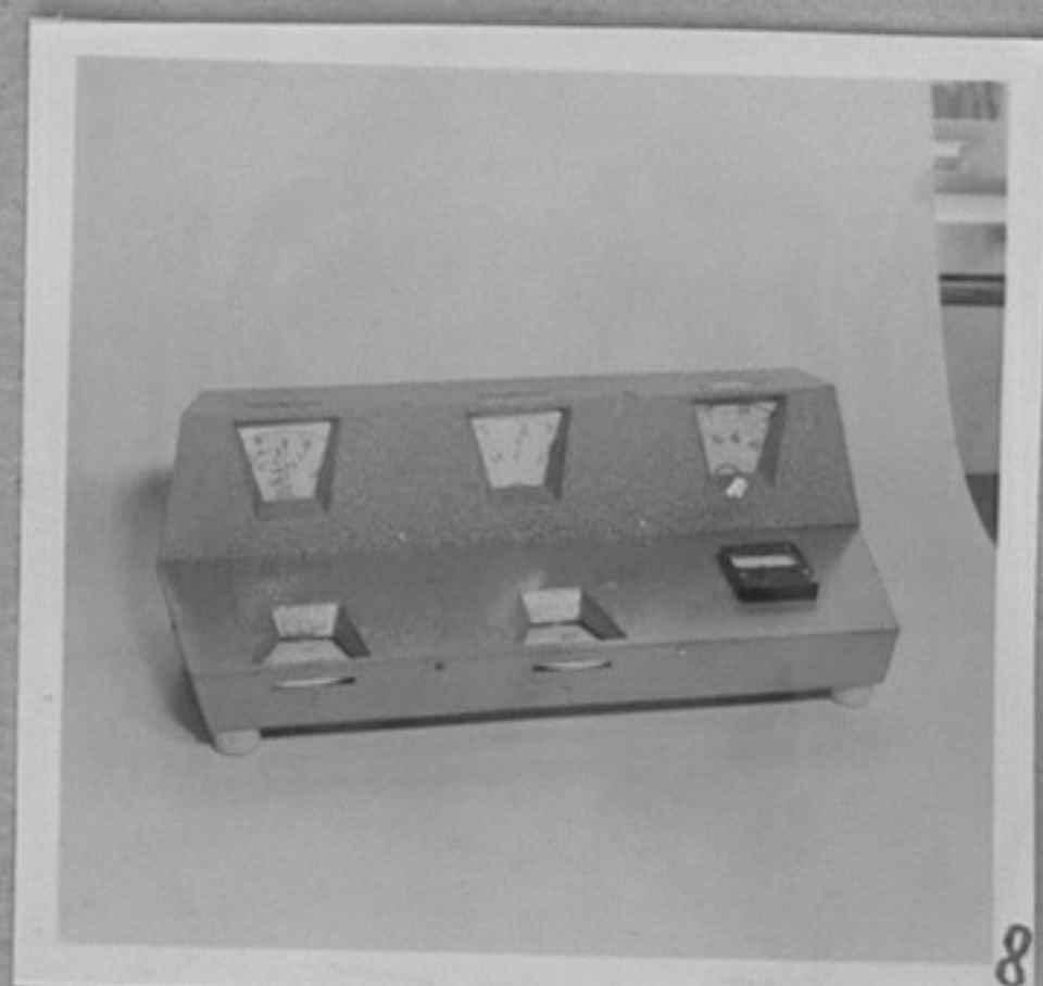
70-367-8-Действащ модел на аналогова изчислителна машина, кръжок "Радиоелектроника". /В.Иванова/ ИК
