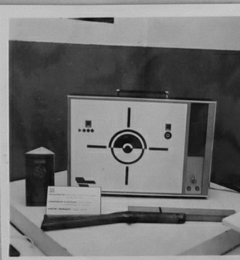
73-4805-1-Електронно портативно стрелбище; авт.колектив -ксер К.Спиртов, Ст.Загора/Из VI-я преглед на ТНТМ в Пловдив/. /Нед.Чобанов/ СС
