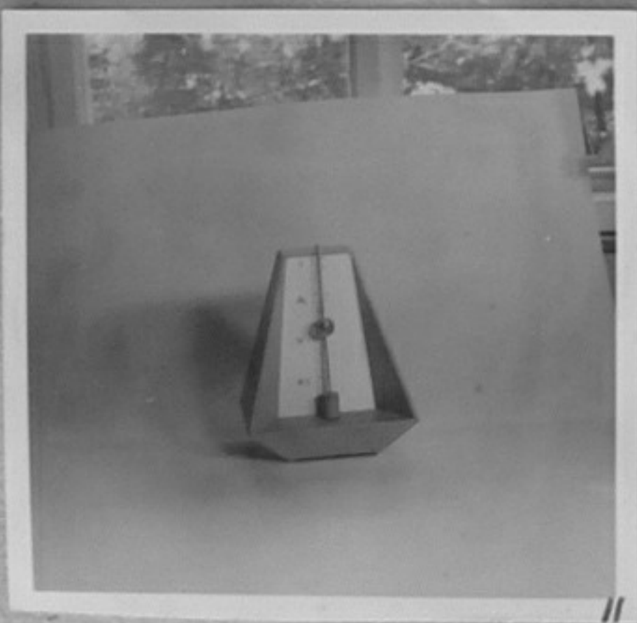
70-367-11-Електронен транзисторен метроном, изработен в кръжока по "Радиоелектроника". /В.Иванова/ ИК
