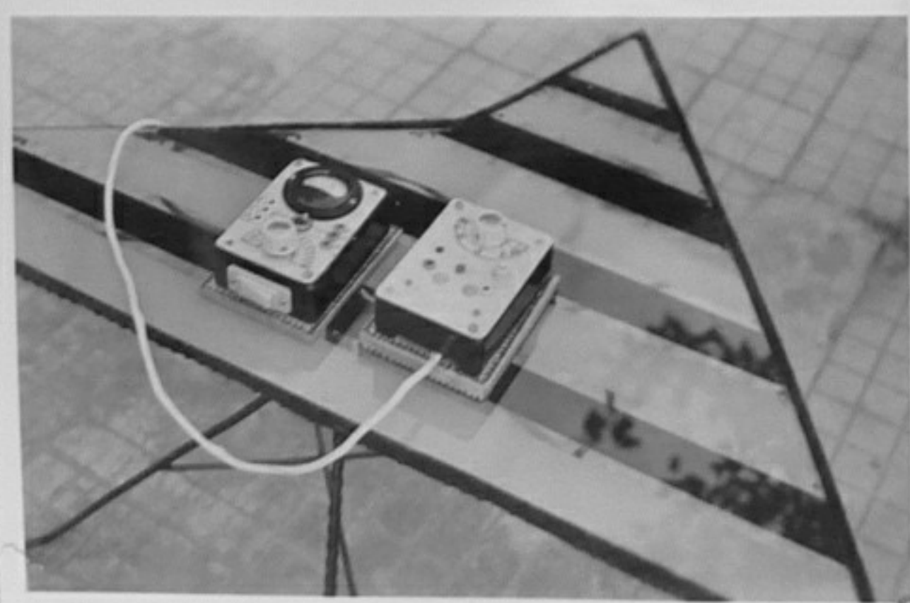
70-3833-2-Уред за измерване на транзистори, изработен от кръжочници по радиотехника в гр.Самоков. /Т.Симеонов/ ИК
