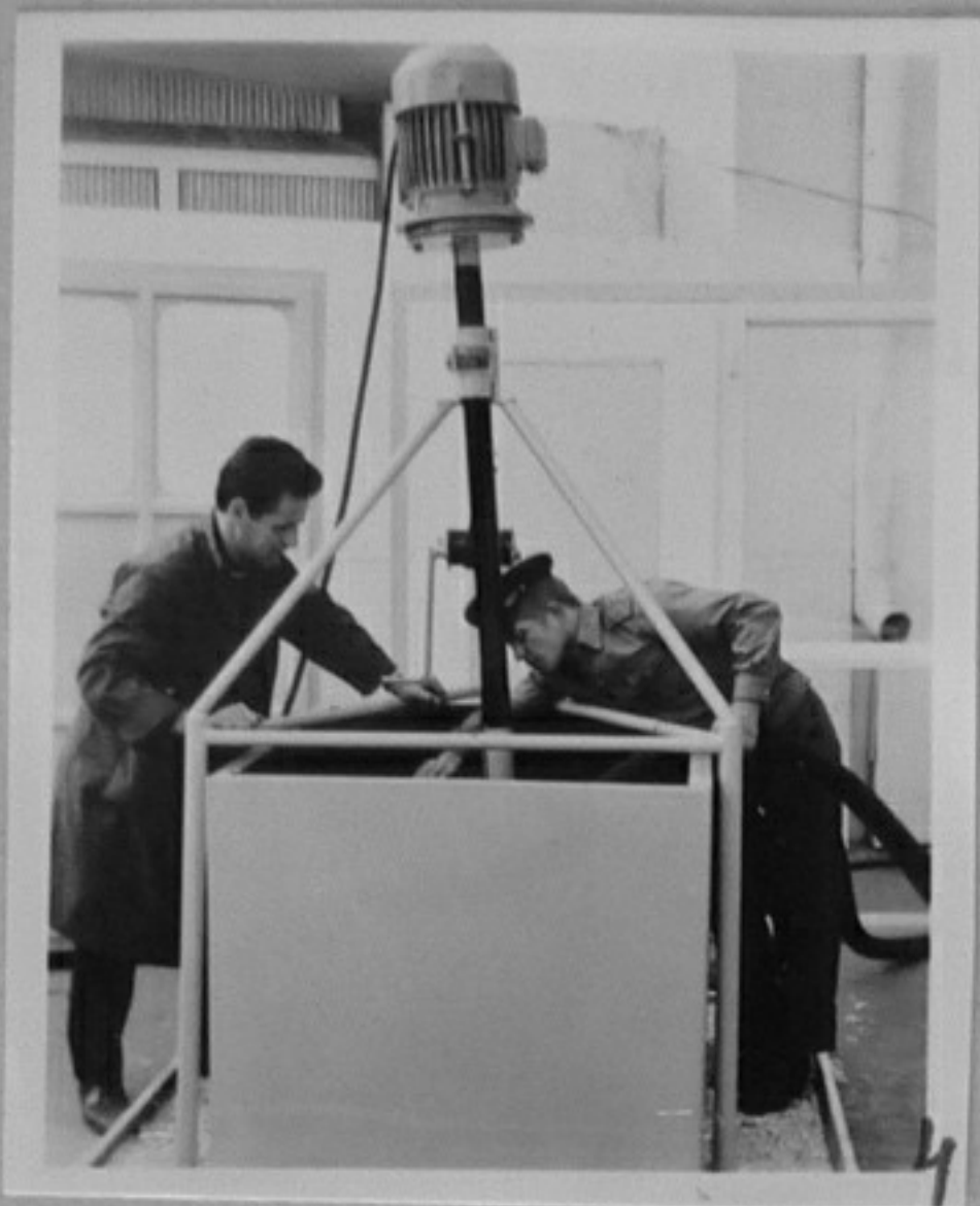
73-4767-4-Устройство за вадене на вар от варници; авторски колектив с ръковод- Симеон Серафимов от под. 30-20. /Нед.Чобанов/СС
