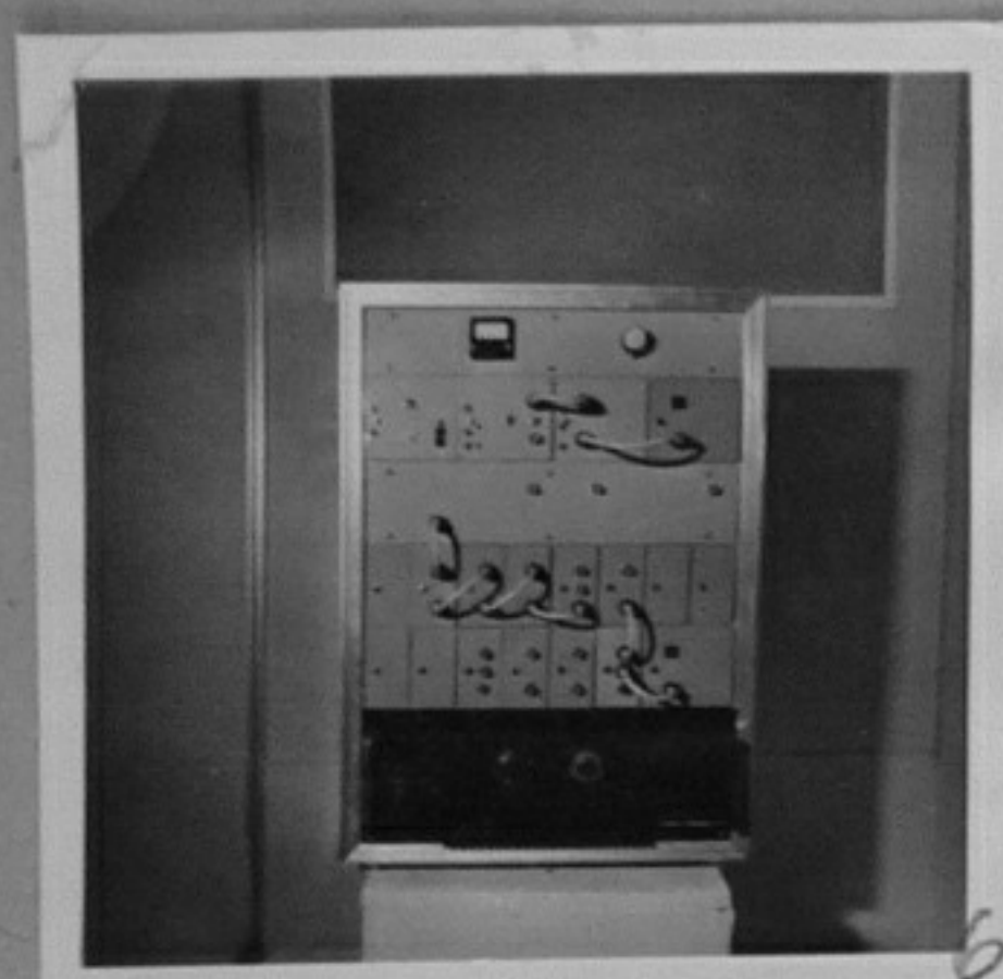
79-3848-6-TV модулятор, разработка от младежки колектив на НИОС-София. /Е.Богоев/АШ
