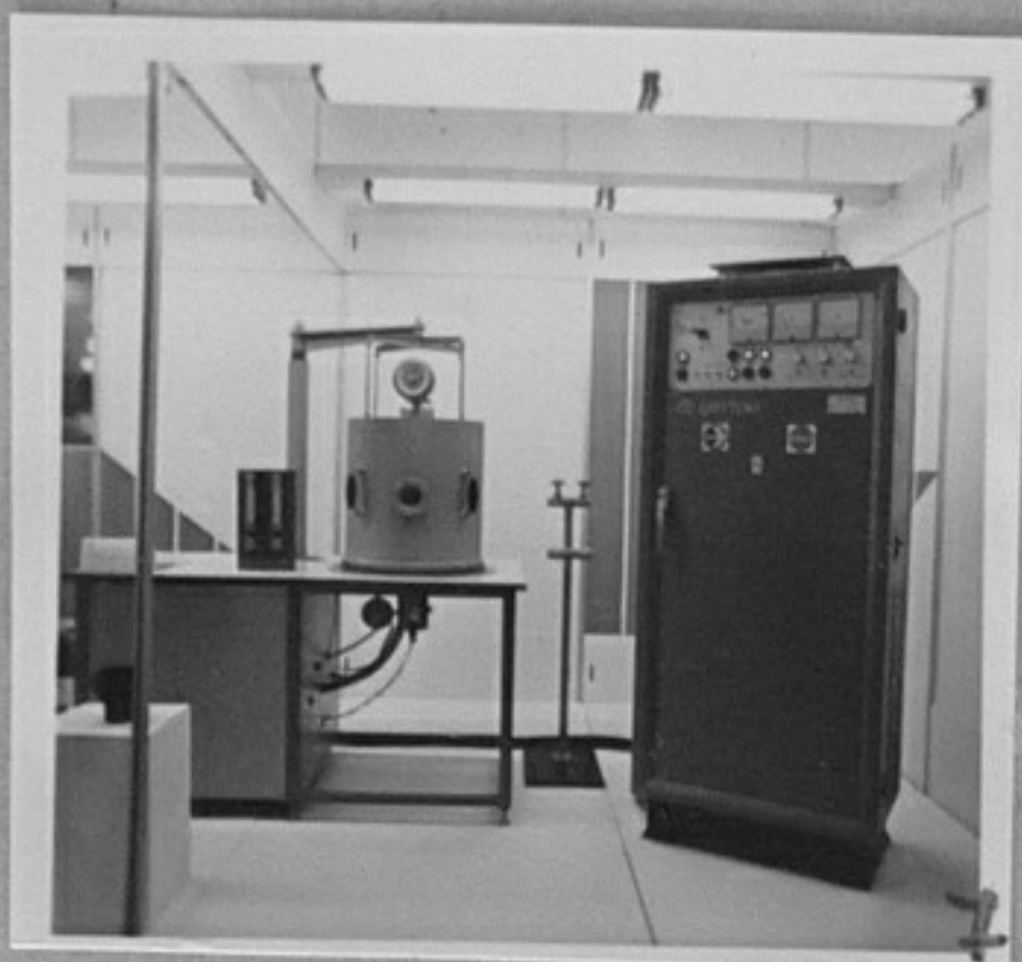
79-3851-7-Клуб при ВМИ "Ленин". Инсталация за химическа термична обработка в електр. тлеещ разряд на метали-йон 15. /Е. Богоев/АШ
