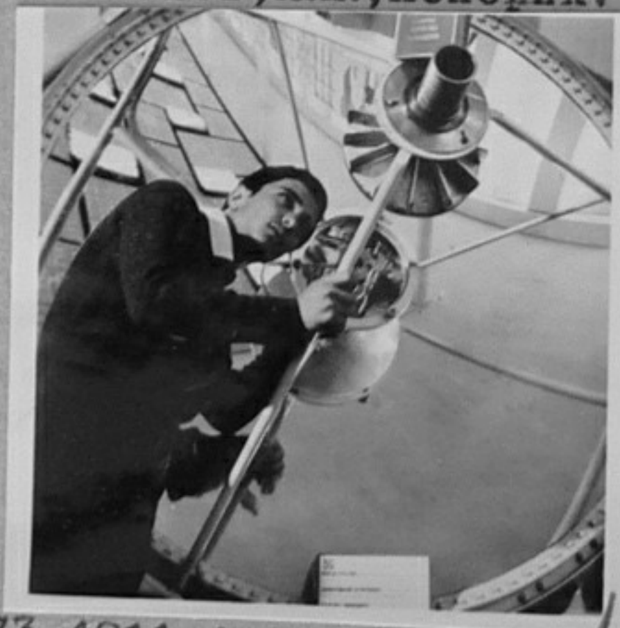
73-4811-1,2-Оптически квантов генератор, захранван от слънчева енергия. Авторски колектив с ръководител - О. Читакия, Бургас.
