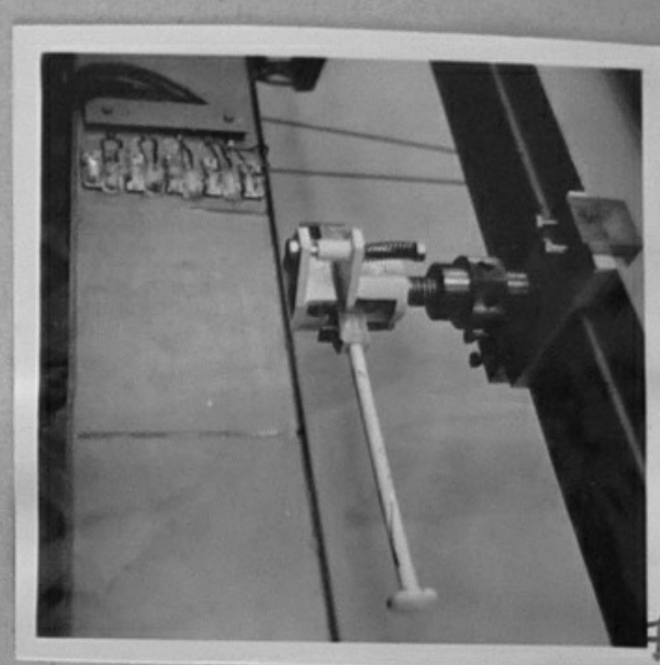
76-591-7-Устройство за вне- запно разтоварване на крано- ви греди, разработка на Н.Ива- нов, гл.асистент Пл.Ексаров и дипломанта Дилян Кожухаров. /В.Иванова/ИК
