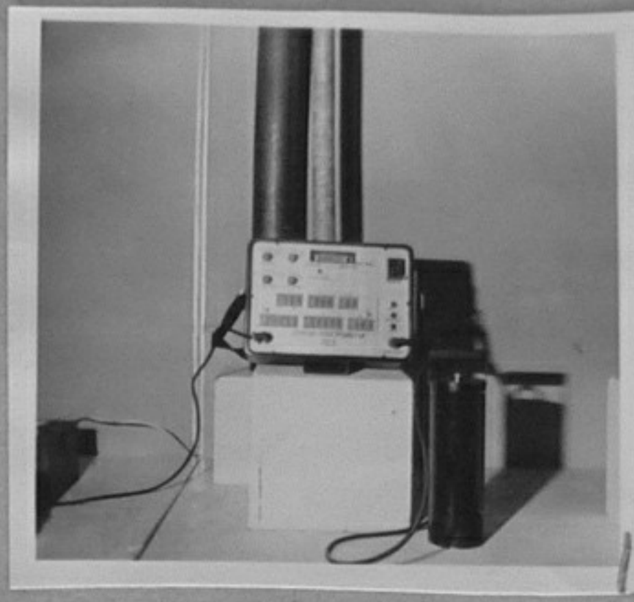
79-3847-1-Полеви триканален гама-спектрометър. /Е.Богоев/АШ
