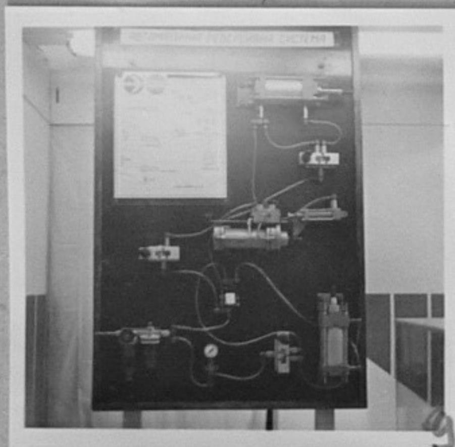
79-3851-9-Пневмозадвижване на машина за гранулиране на разтворимо кафе. /Е. Богоев/АШ
