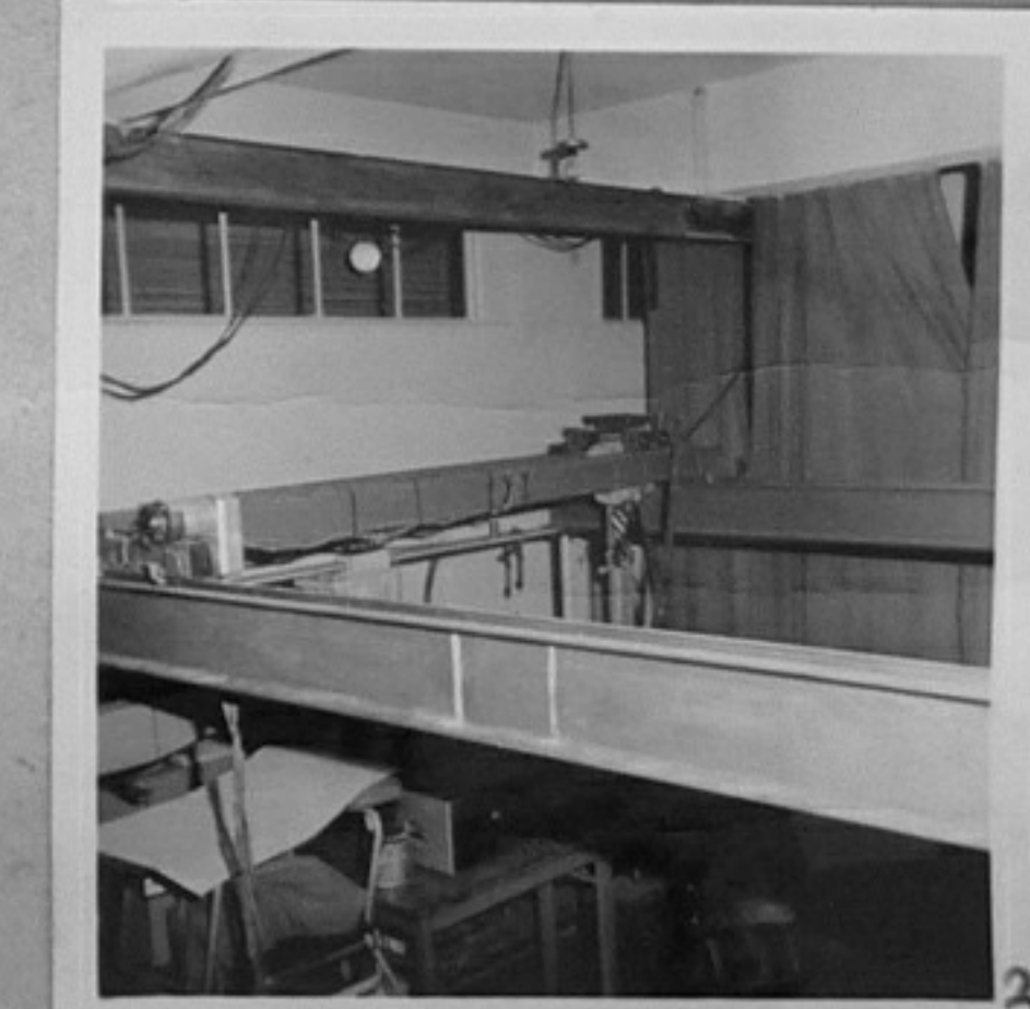
76-592-3-Мостов кран с про- менлив отвор, разработка на гл.асистент Пл.Ексаров и инж.Чавдар Здравков. /В.Иванова/ИК
