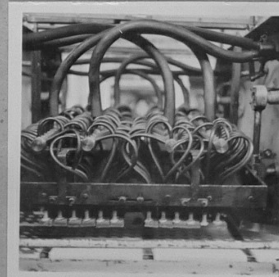
76-1225-7-ЗШИ "Република"-Своге. Автомат за нареждане на плътни бомбони тип "Хайденау". Ян.Лозанов и Мл.Аспарухов по време на работа.
