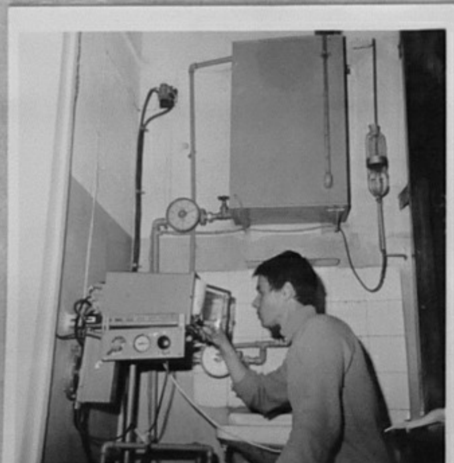
76-593-2-Студентът от IV курс Делчев Вичев работи на установка за моделиране и изследване на хидравлични обекти. /В.Иванова/ИК
