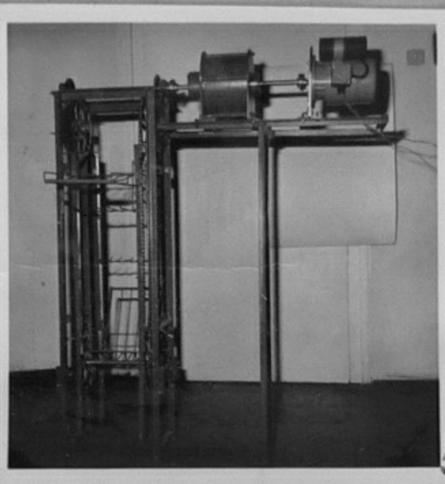
76-591-5-Елеватор с въл- нова предавка, разработил гл.асистент Н.Иванов. /В.Иванова/ИК
