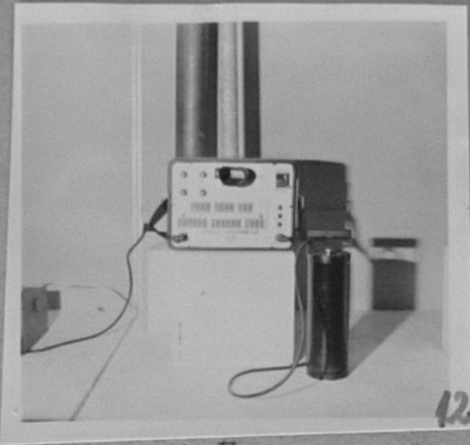
79-3846-13-Полеви триканален гама-спектрометър. /Е.Богоев/АШ
