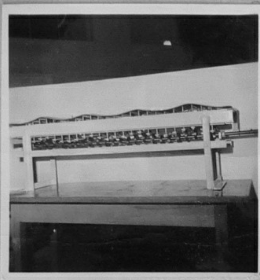
76-591-3-Вълнов транспор- тор, разработил колектив с гл.асистент Н.Иванов. /В.Иванова/ИК
