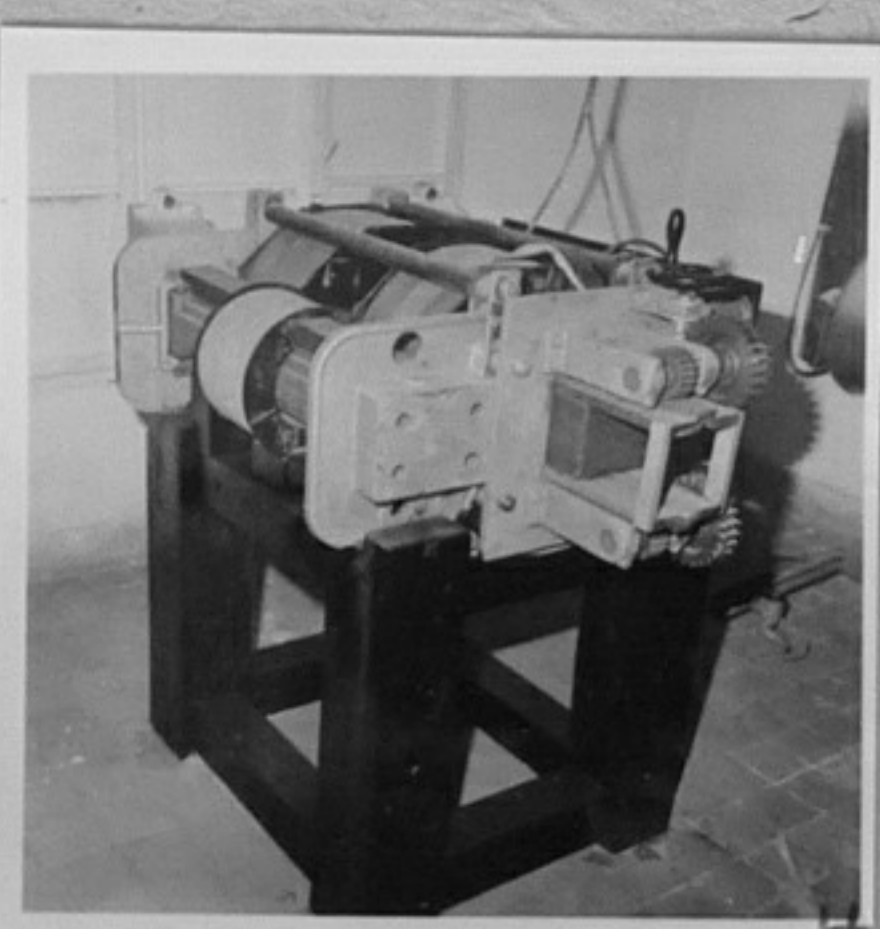
Обекти на ТНТМ-София. Висш машинно-електротехнически институт. /В.Балевска/ИК 76-612-10-Асистентът Чобанов и студентът Л. Маринов по време на упражнението по изучаване на технологичните възможности на стан АТПК за прокарване на повече вътъци едновременно. /В.Иванова/ИК 76-613-4-Електромагнитна установка за въздействие върху леснотопими метали сплави, разработил колектив с ръководител Вл.Христов. 76-613-5-Кръжочникът Димитър Атанасов по време на занимание.
