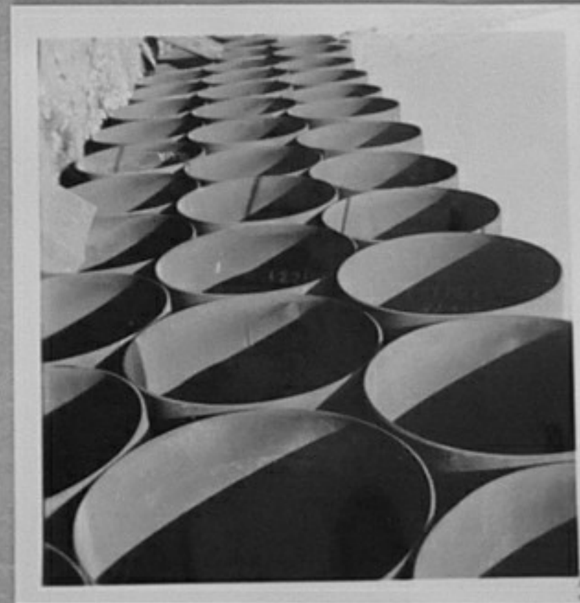
Газопровод СССР-България. База за автоматично заваряване на тръби за газопровод и вода, в с. Тодорово, Плевенски окръг. /Л. Златков/ МК 72-1637-2-Съветският специалист по заварките Б. Оболенски дава инструктаж на работници от базата. 72-1637-5-Тръби за газопровода. 72-1637-10-Газорезещата машина "Спътник" за автоматично отрязване на тръбите се настройва от комсомолец Георги Борисов.
