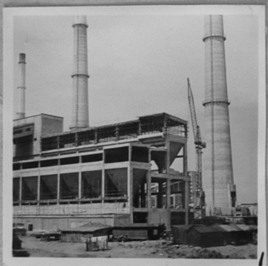
68-3683-1,2,3 - Разширение и строеж на нова сушилна фабрика при ТЕЦ-2 от комплекса "Марица изток", с.Ковачево, Сливенски окръг. /Кр.Арсов/ ЕИ
