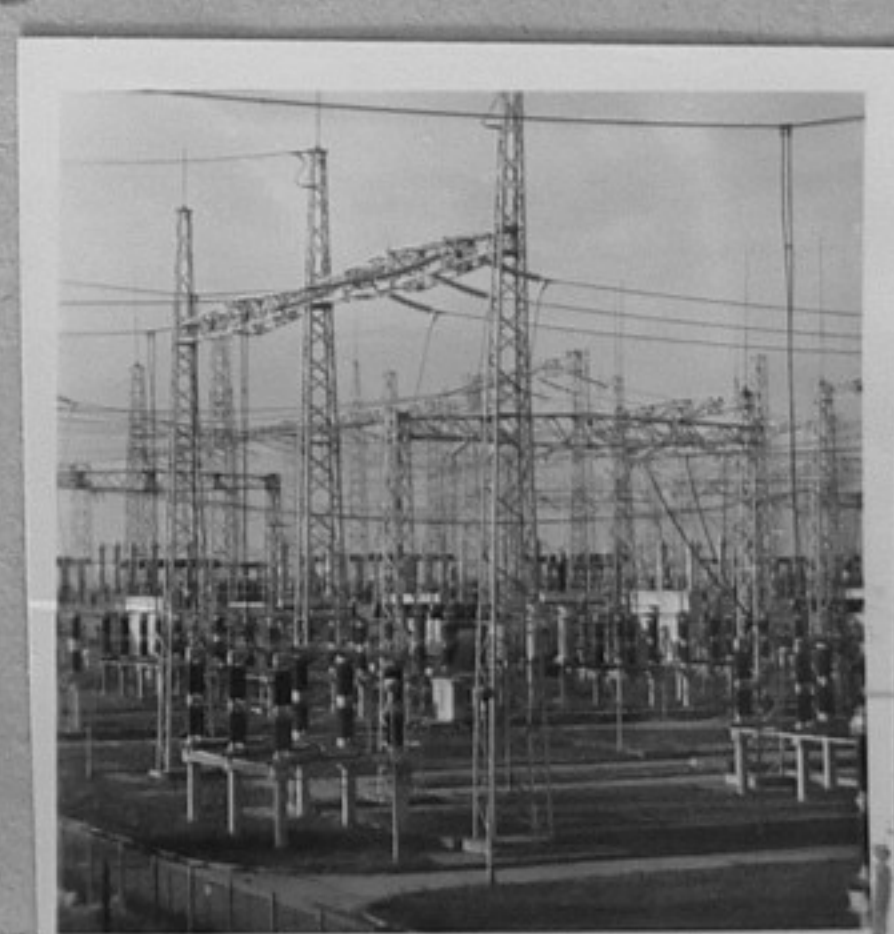
80-3756-1-Съоръженията на откритата разпредели- телна уредба. Р. Марукян/АШ
