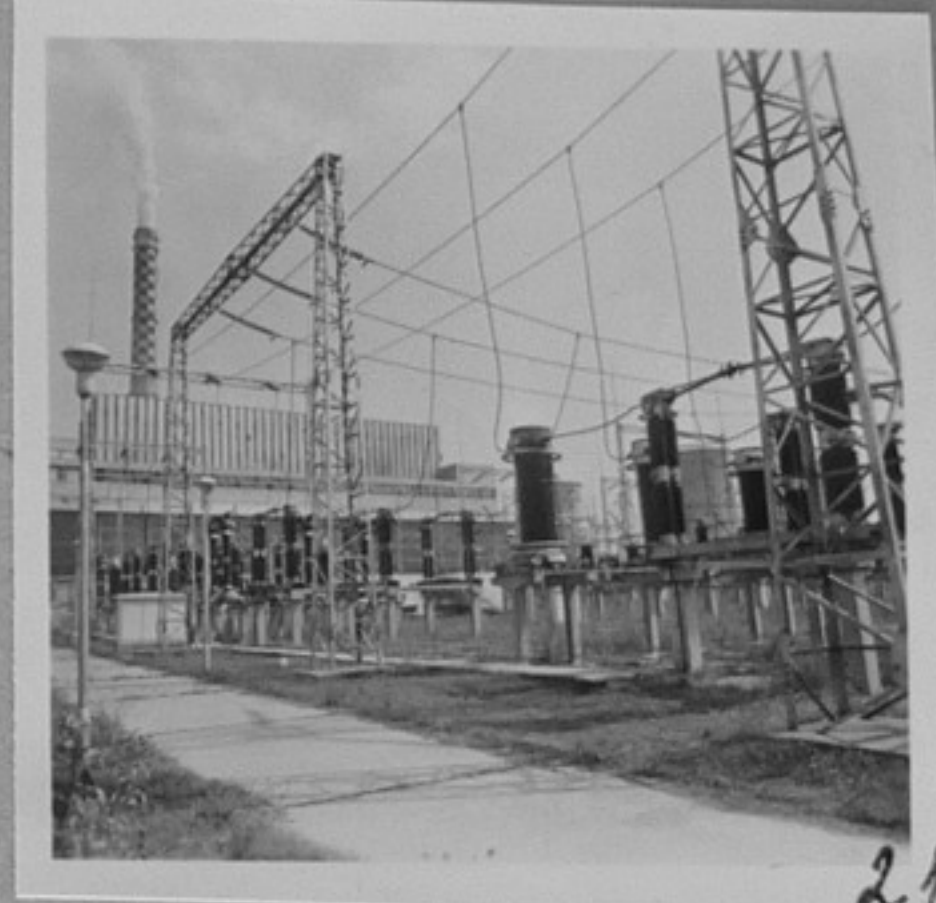
78-2607-17,21-Разпределителна станция в Бобов дол. /Е.Киров/АШ
