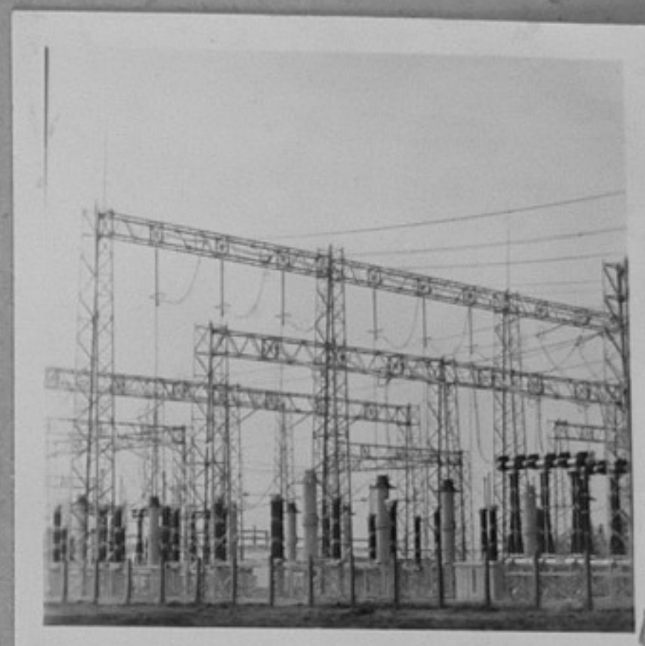
81-1725-1-Ел. подстанция край Бургас. В. Балева/АШ
