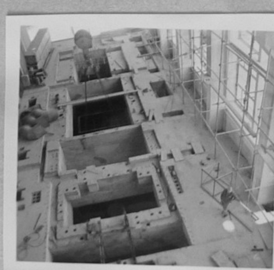
70-2343-4-Извършва се разширение на турбин- ната зала. /П.Божков/ ХП
