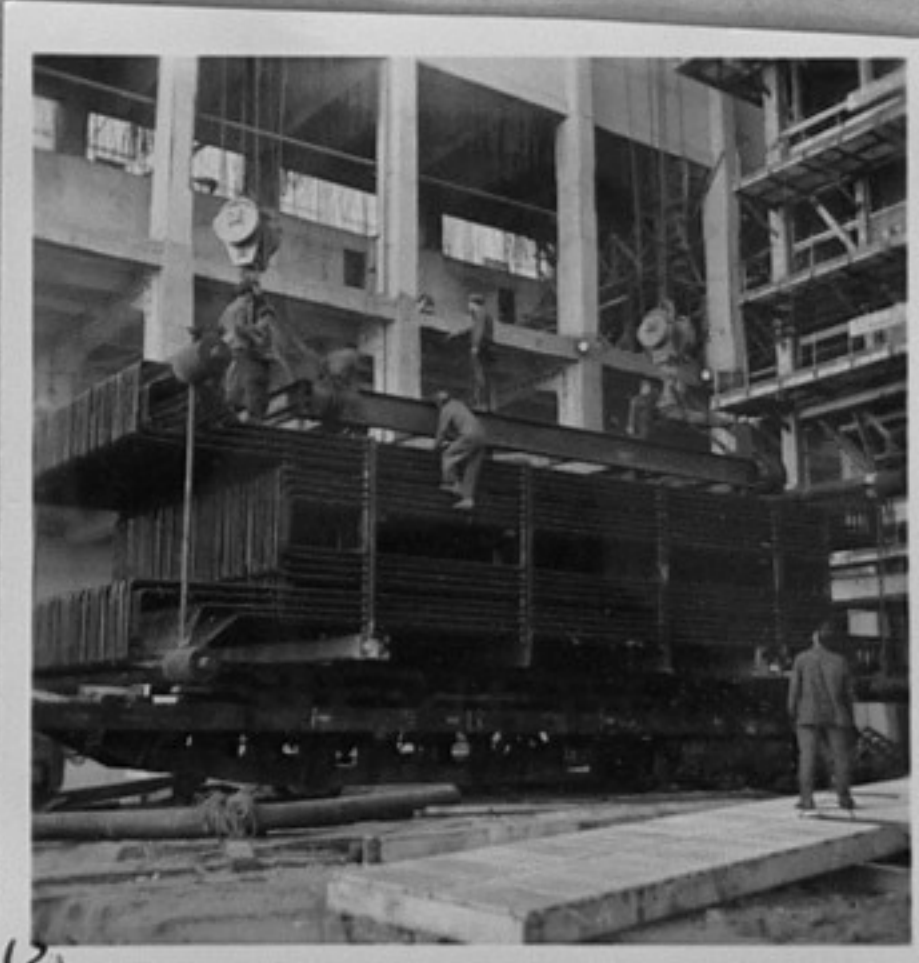
62/2564-12-Пренасяне на паропрегревателя I-ва степен на 7-ми котел при ТЕЦ. /Иор- данов/ ММ
