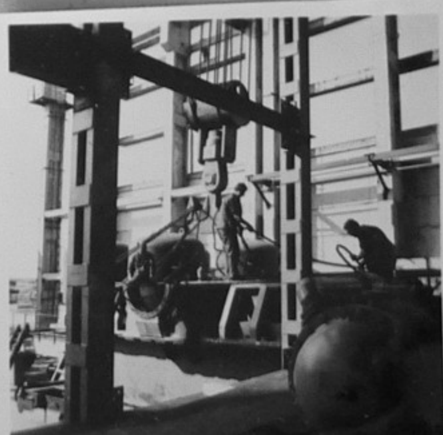
8 - Долна половина на цилиндъра с ниско налягане към турбинния цех.
