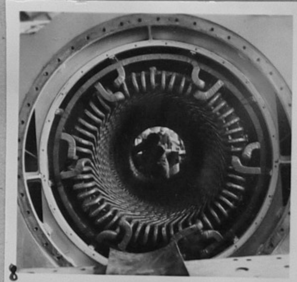
65/707-5,7,8 - Монтаж на втора турбина - работи бригадата на Крум Славчев. /Парушев/ ММ
