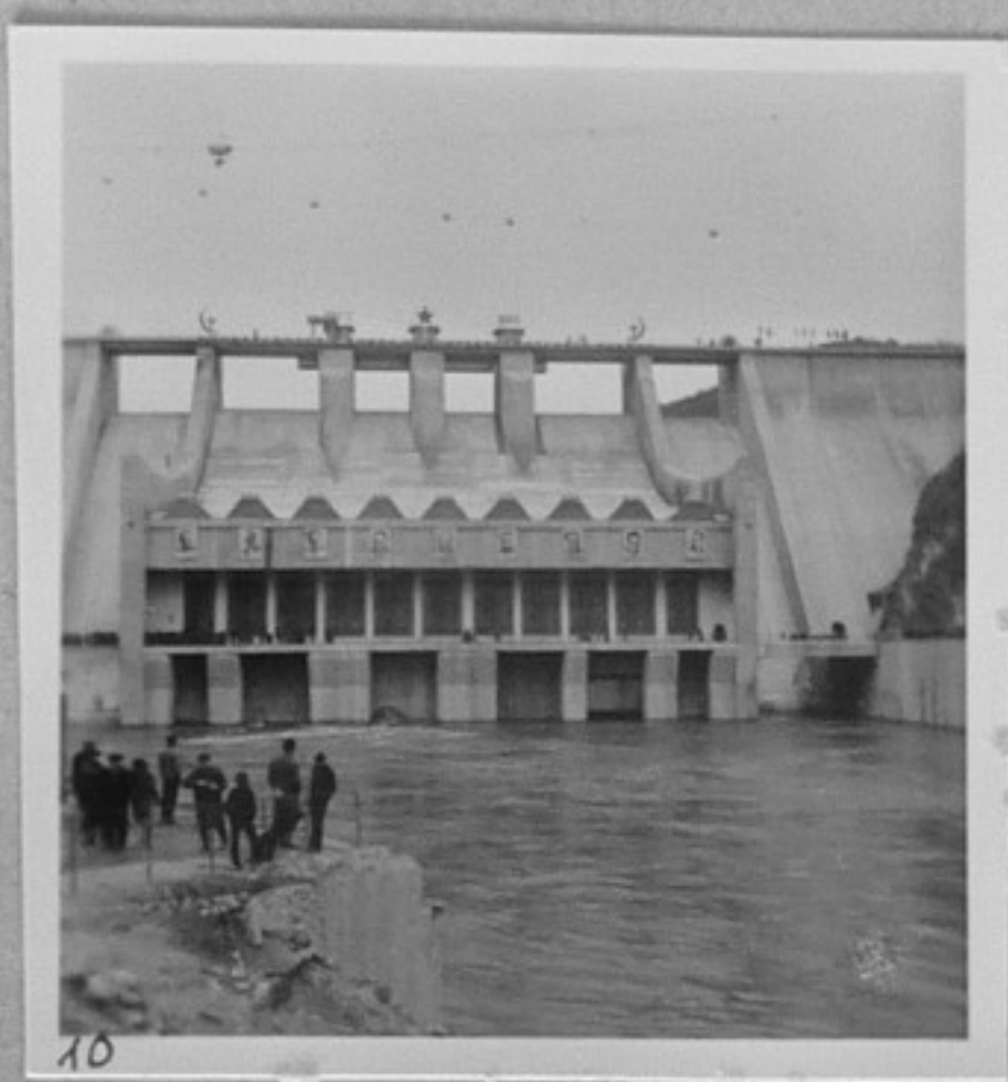
64/3522-8,10 - Общи изгледи на ВЕЦ. /Ангелов/ ММ
