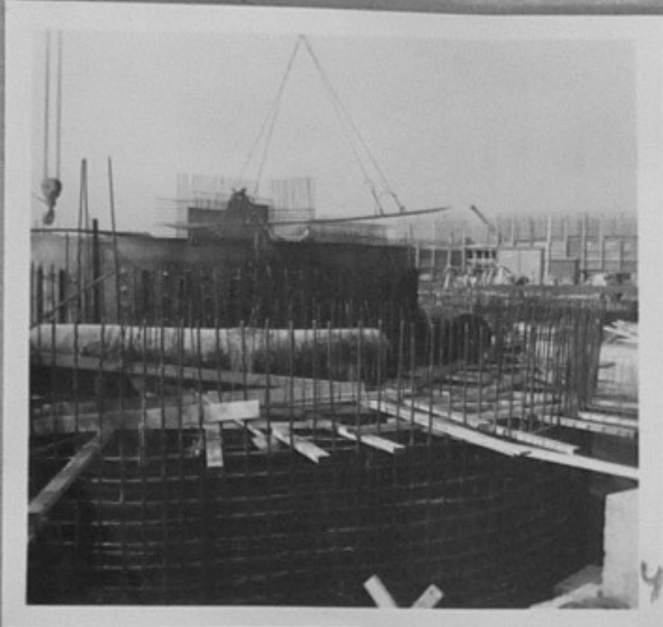
71-665-2, 4, 11-На строежа на първия атомен реактор. /Л.Златков/ XII
