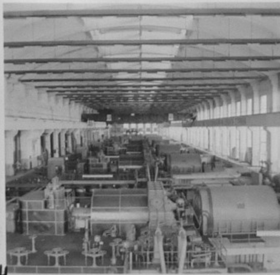
64/2322-2,4,6 - Турбо-генераторната зала. /Божков/ ММ
