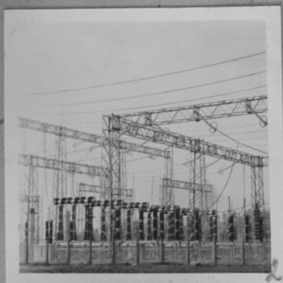
81-1725-2, 3, 4-Подстанцията край Бургас.
