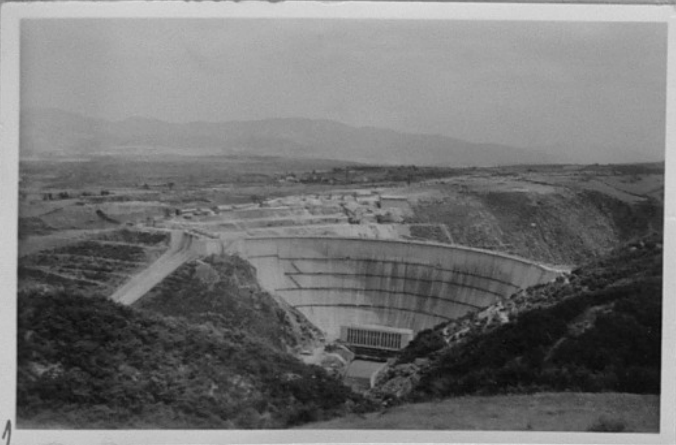
64/1980-1-Общ изглед. /Янев/ ММ
