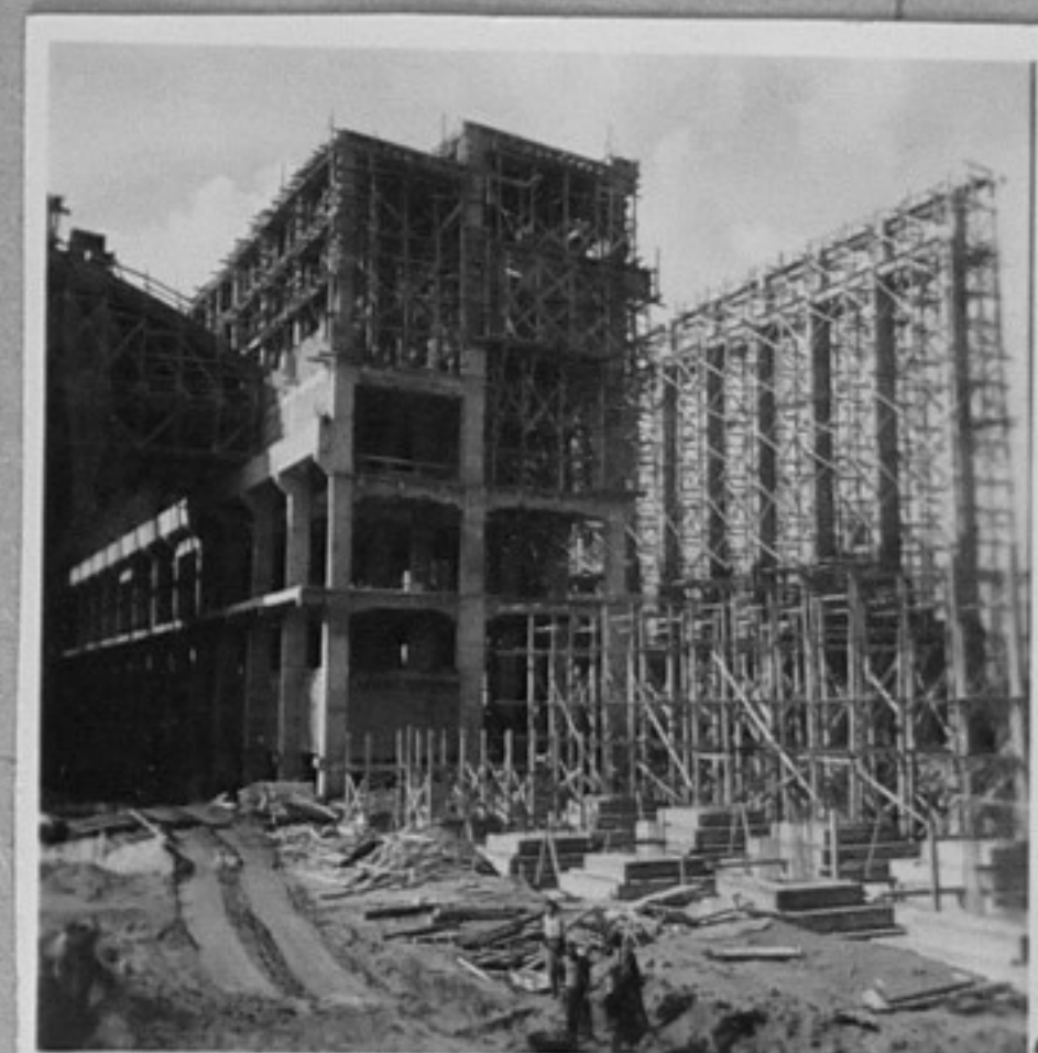
59/1009-2- На строежа на ТЕЦ "Марица изток". /Кожухаров/
