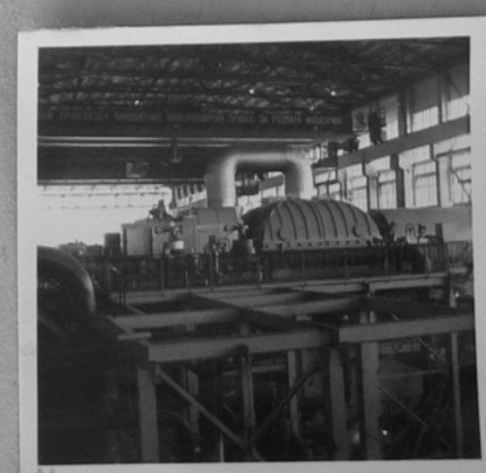
67-3473-11-Втора турбина- пусната в действие м.юли 1967 година. /Кр. Арсов/СС
