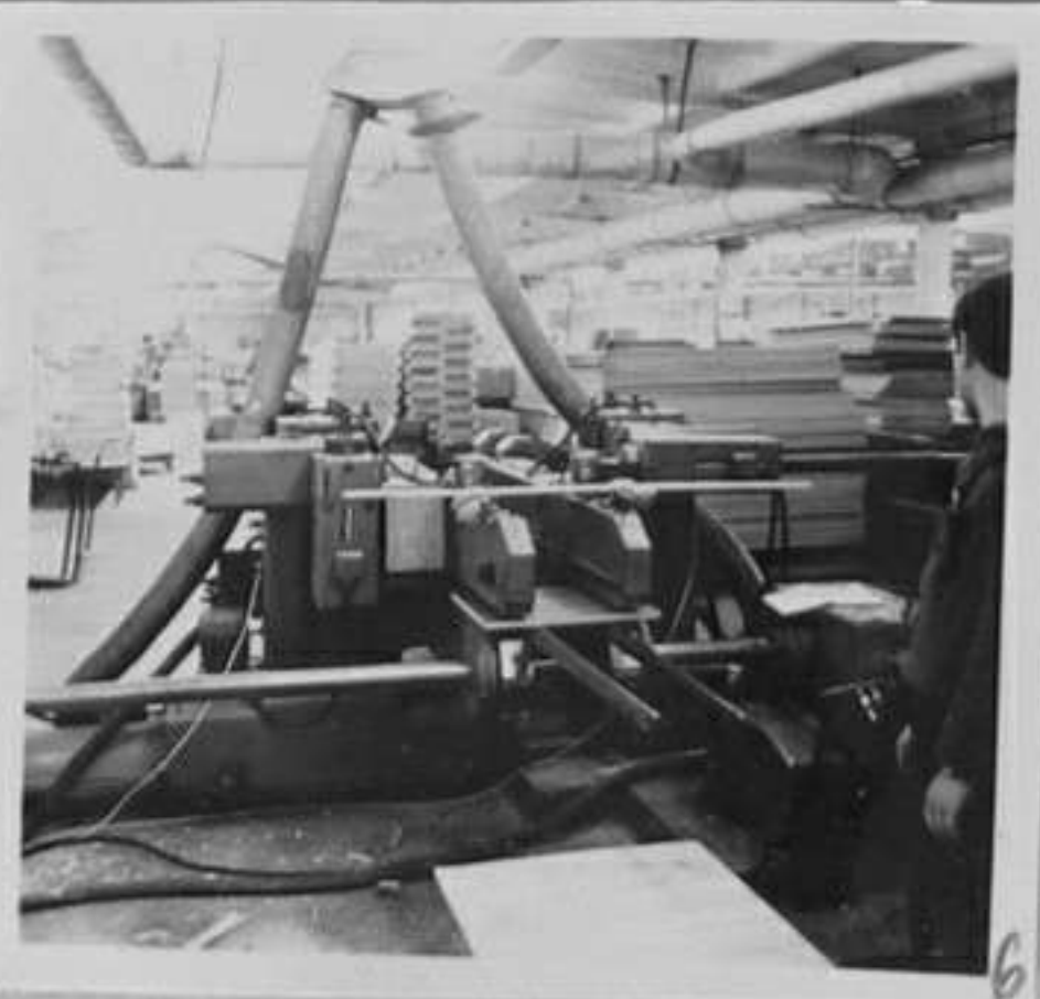
72-5551-5,6-Многооперационен агрегат за точна машинна обработка "Челоски". /Н.Чобанов/ИК
