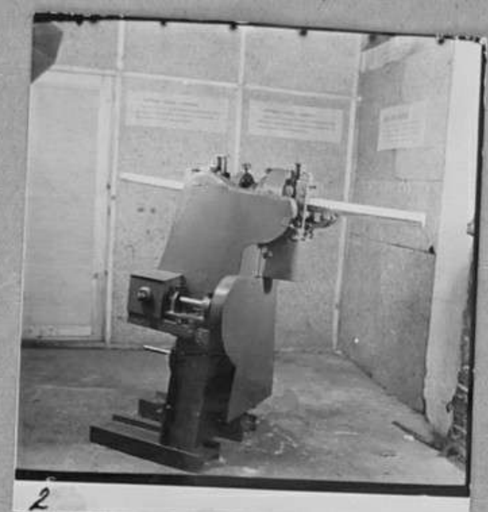
1,2 - Автоматична бусола за изработване части на столове, обслужвана само от 1 работник.
