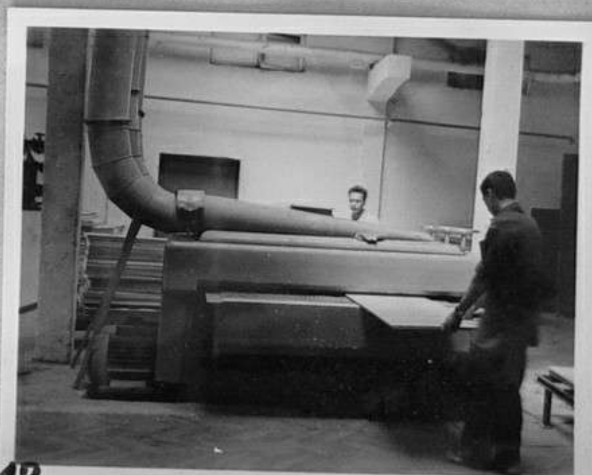
67-2737-10- Шлайфане на фурнирвани плоскости. /Димитър Сибирски/СС
