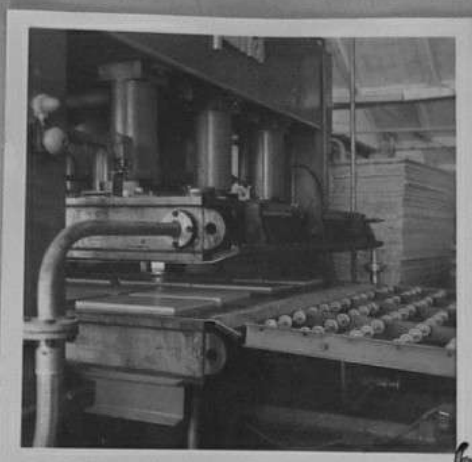
68-4613-6,7-Излизане на готовите плоскости от пресата след залепване. /Д.Рогев/ XII
