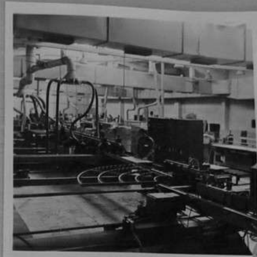
79-2795-6 Автоматична линия в завод "Добруджанска мебел", за лепене на фурнир към плоскостта Е.Киров/МД
