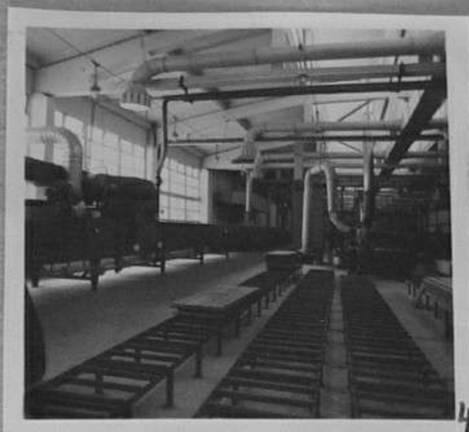
73-3063-4-Лакоразливна линия. /В.Иванова/ТК
