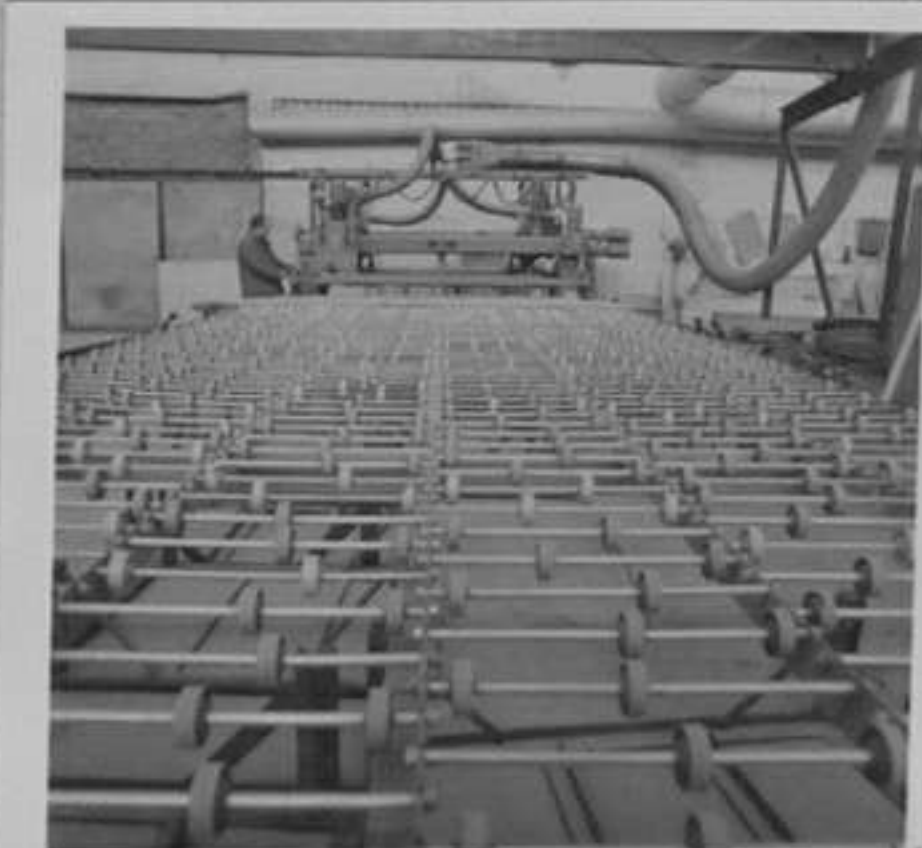
78-3868-4-Форматно об- рязващ циркуляр. /Х. Румян/АШ
