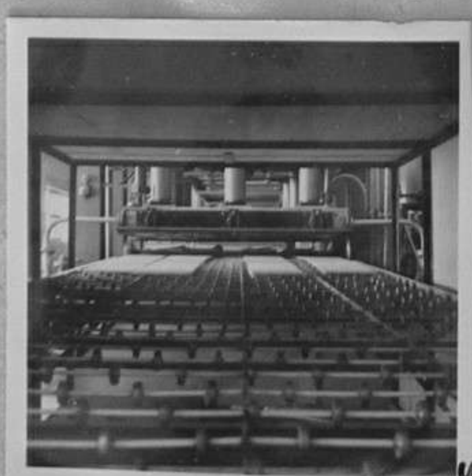
68-4613-4,5-Излизане на готовите плоскости от пресата след залепване. /Д.Рогев/ XII
