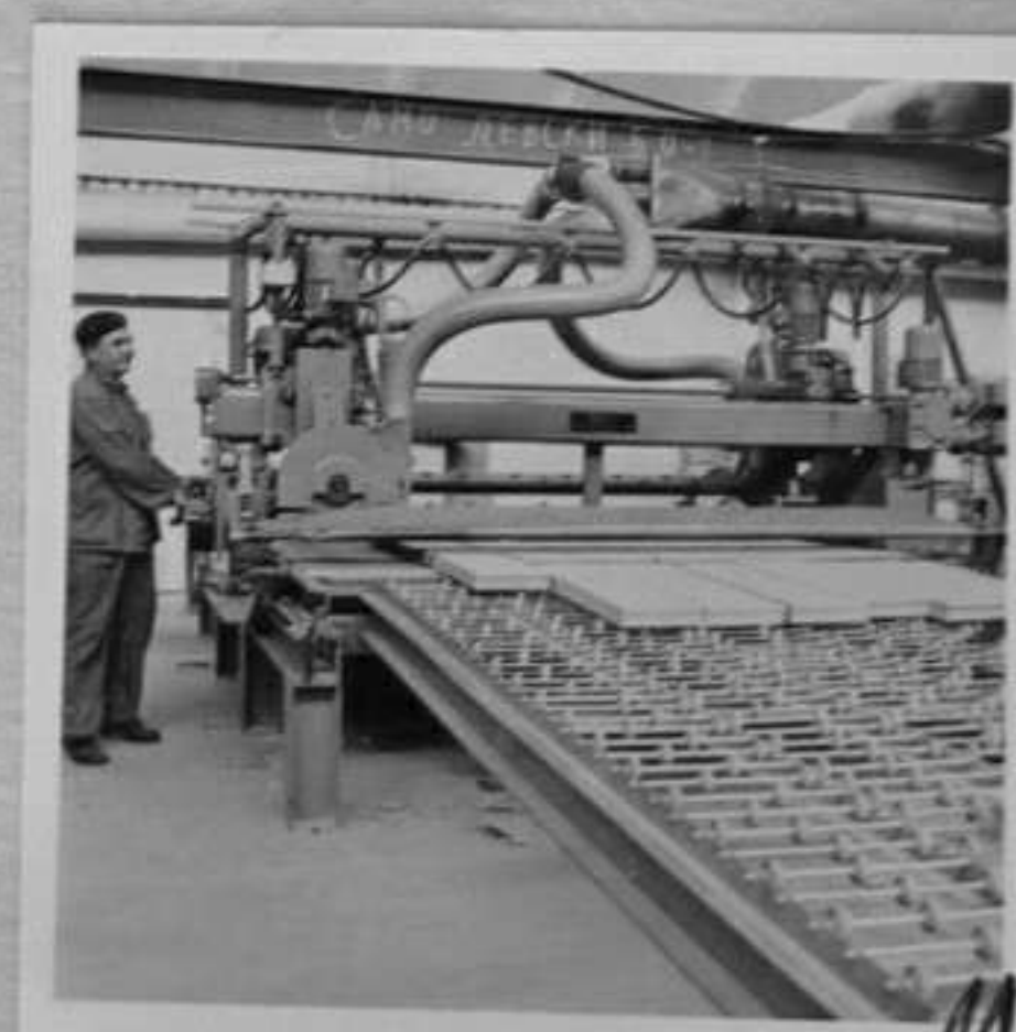
77-2322-11-Автоматичен станциг за разкрояване на плоскости с програмно устройство. /Р.Марукян/ЛА
