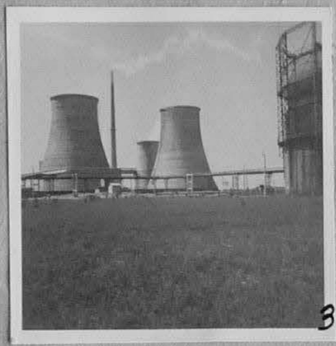
1.- Общ изглед на завода. 3,4 - Охладителните кули.
