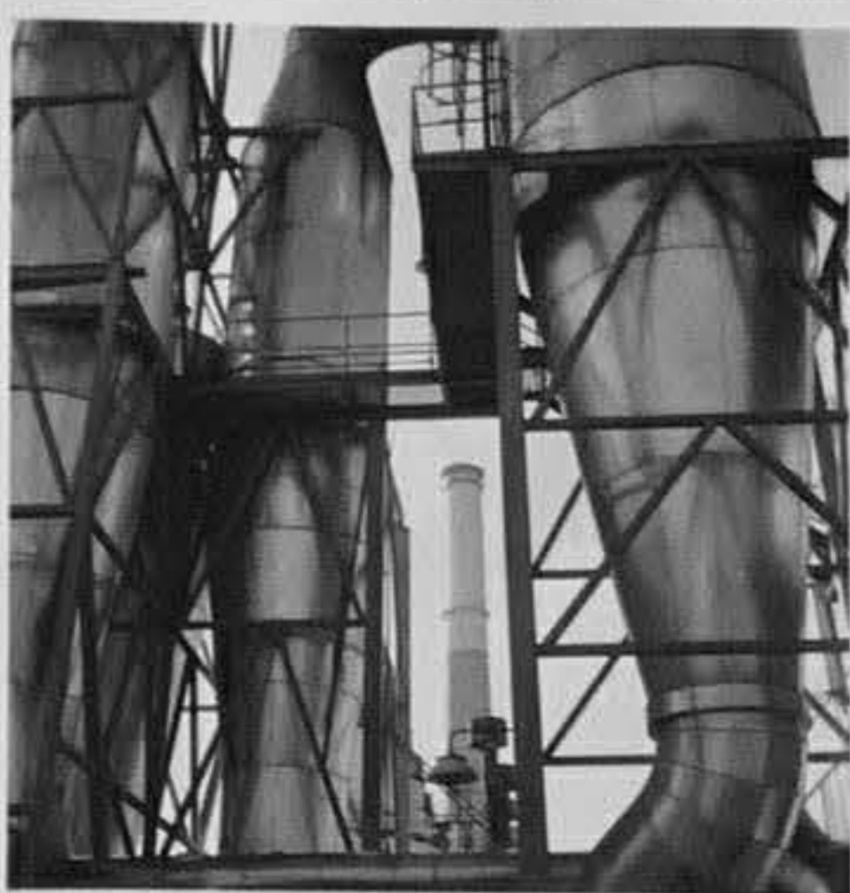
73-4829-2,3-Инсталацията за сушене на целулоза. /Т.Хорисян/ИК
