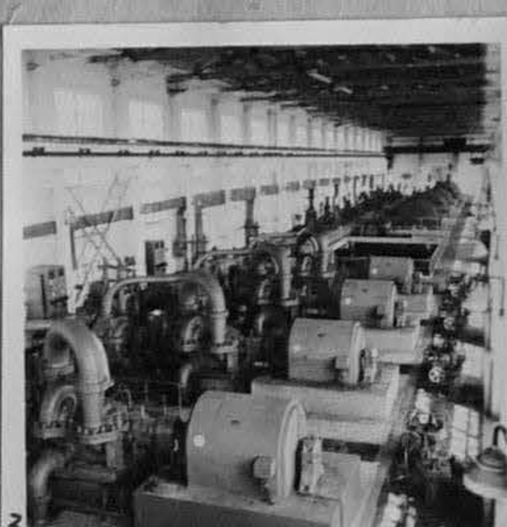
64/1020-3-Цех за синтез на амоняка. /Чаръкчиев/ ММ
