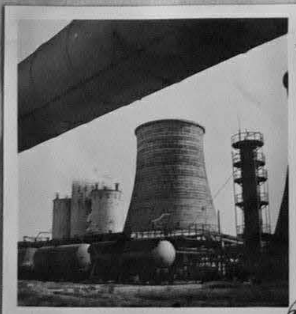
68-4863-5,6-Външен вид на цеха за амониева селитра.
