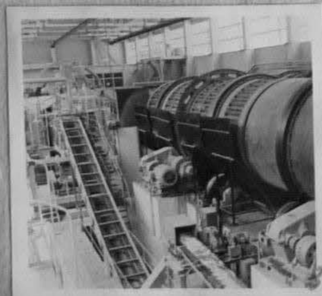
72-3750-3,4-Цех "Каустизация и регенерация" към целулозен завод. /Л.Златков/МК
