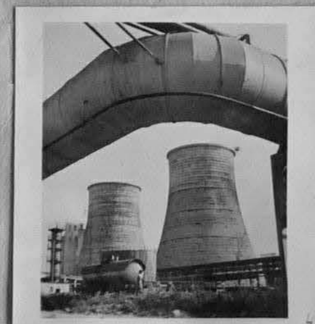
68-4863-3,4-Изгледи от охладителните кули.
