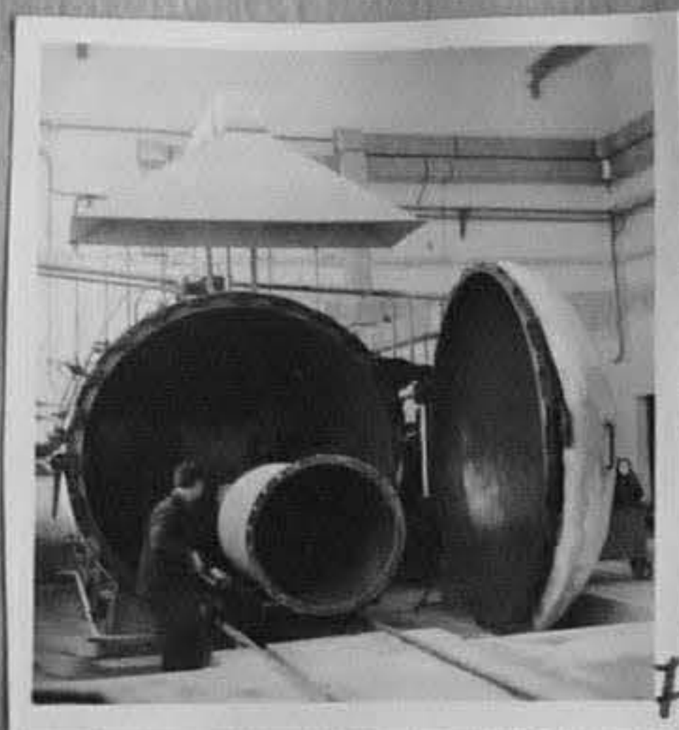
71-664-7,10-В цеха за антикорозионни покрития. /Л.Златков/ ИК
