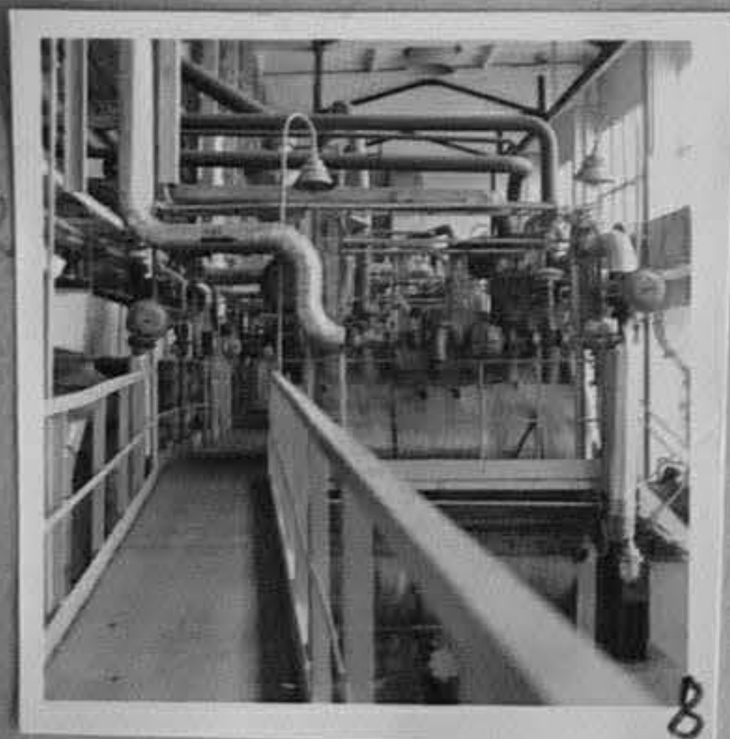
78-2213-8 Химически цех - отделение за ксантогениране Р. Марукян/МД
