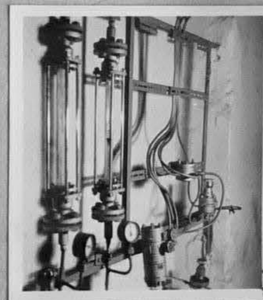
71-257-7-Схема за авто- матично регулиране тем- пературата, газификация на мазутен генератор, из- работена в завода. /Н.Чобанов/ ИК
