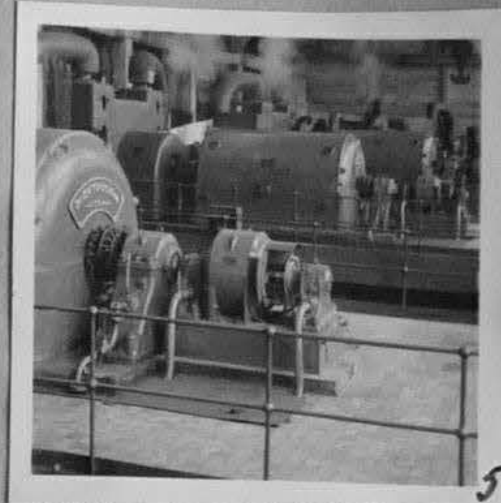
69-967-5-Турбинната зала. /К.Арсов/ ХП
