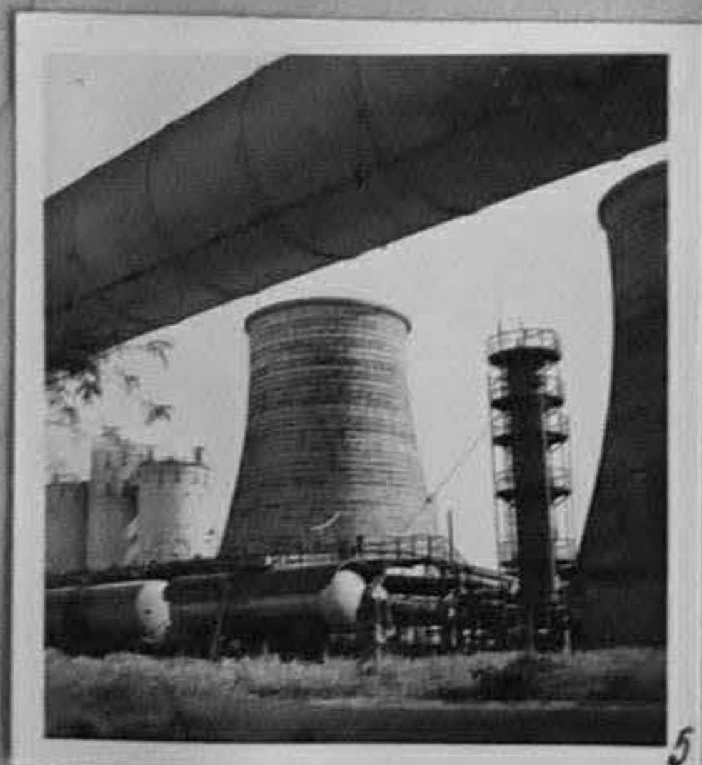
68-4863-5,6-Външен вид на цеха за амониева селитра.
