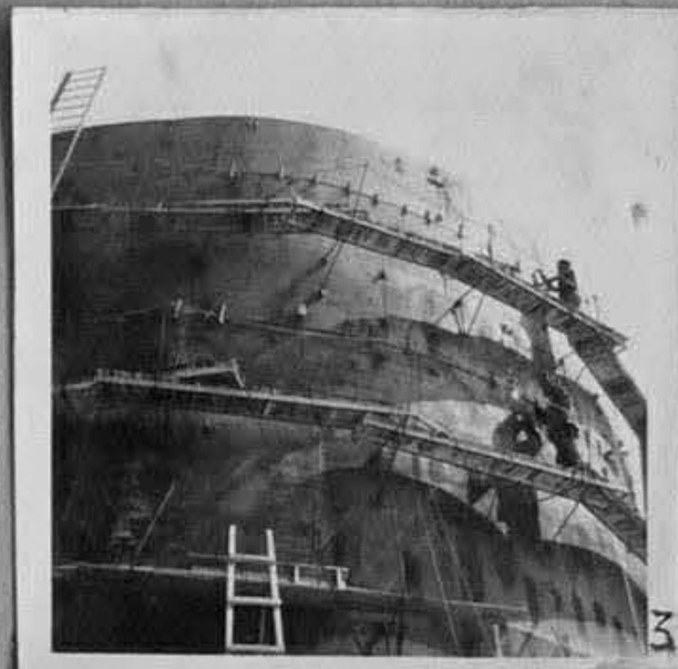
60/2796-3-Резервоара за течен амониак. /Хорисян/
