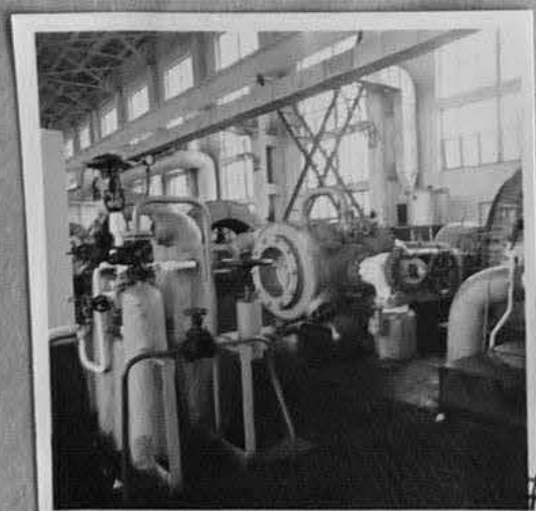
78-361-7 Амониачни компресори в СХК Ст. Загора Р. Марукян/МД
