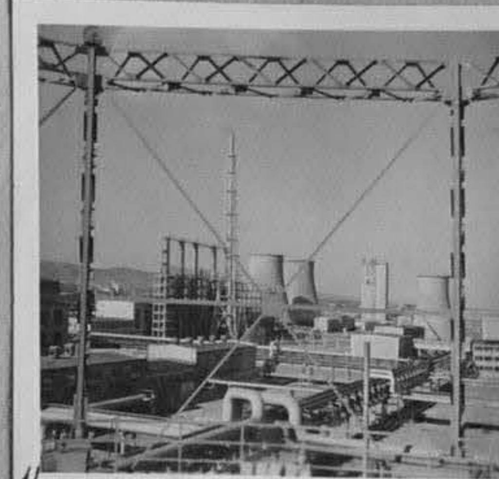
63/1938-7,9,11 - Изгледи от отделните участъци на завода. /Чаръкчиев/ ИИ
