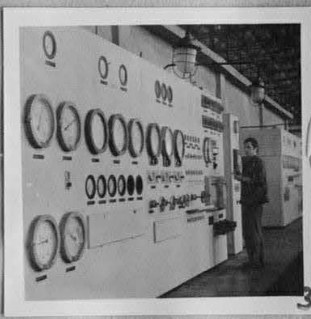
69-964-3,5-Командната зала на цеха за разделяне на въздуха. /К.Арсов/ XII
