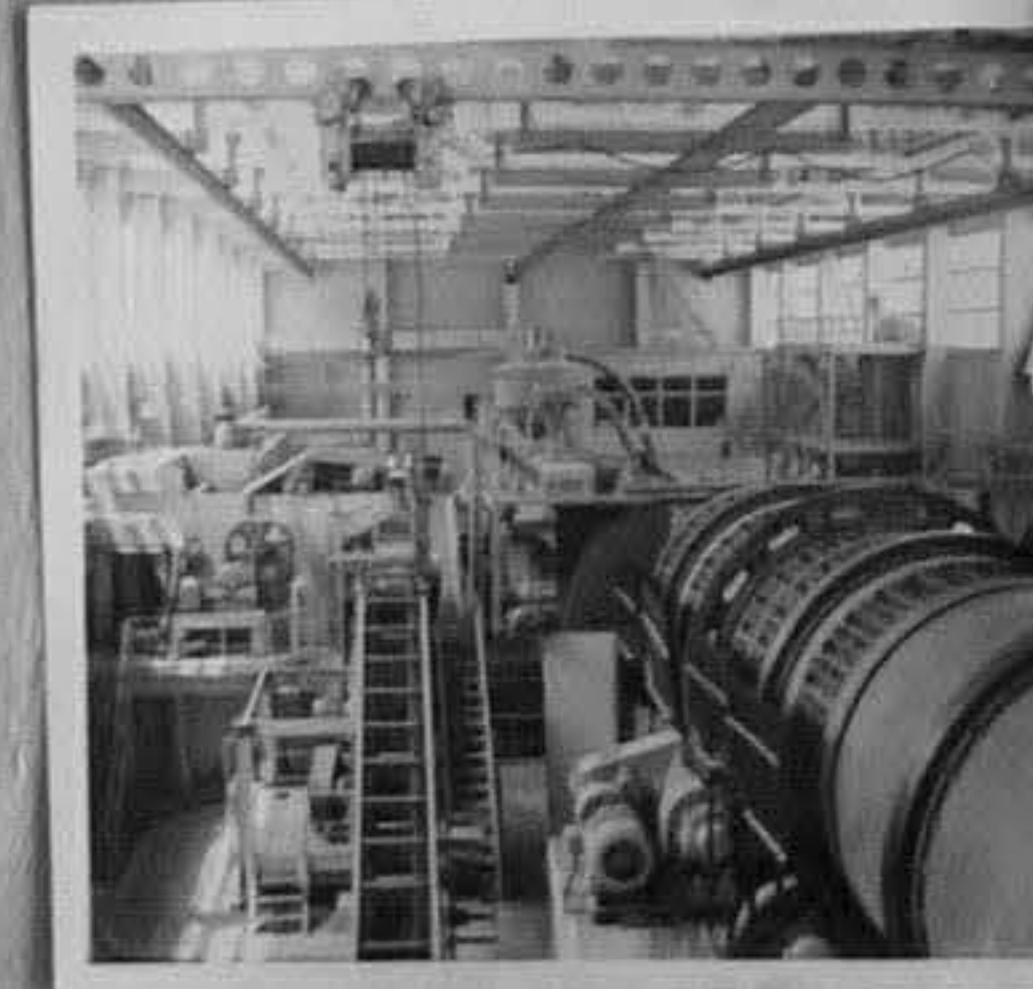
72-3750-3,4-Цех "Каустизация и регенерация" към целулозен завод. /Л.Златков/МК
