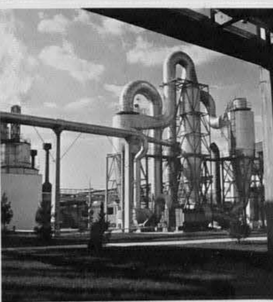
73-4827-8,10,11-Инсталации за сушене на целулоза. /Т.Хорисян/ИК
