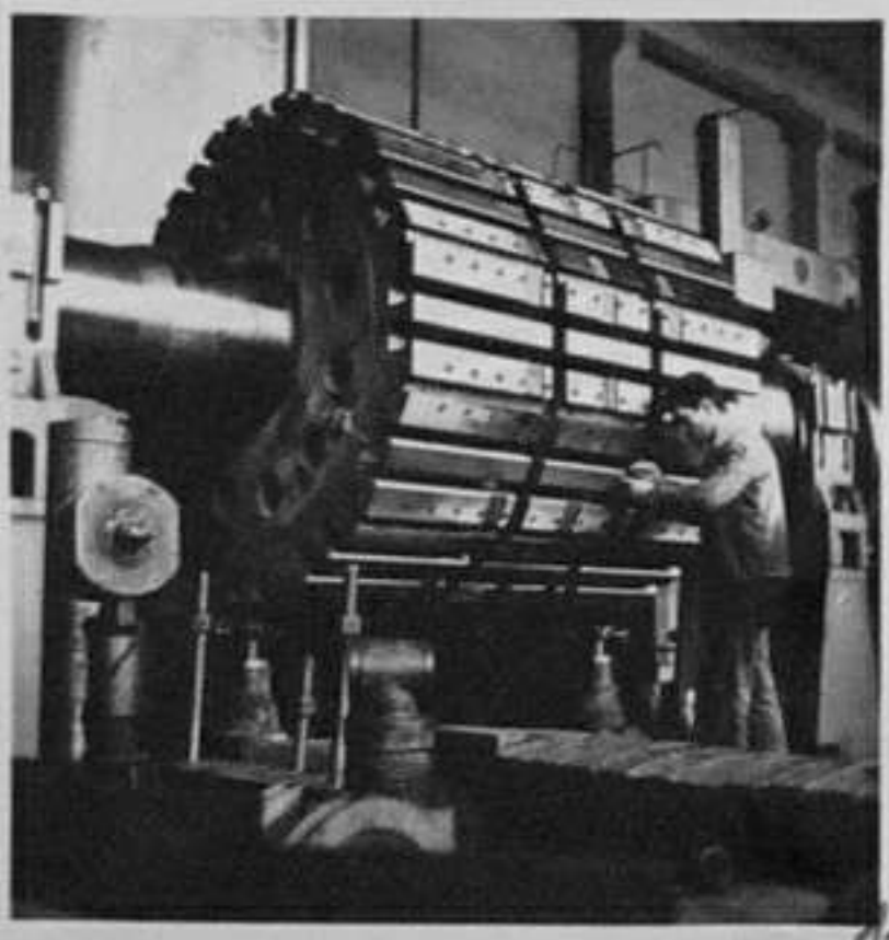
67/523-11,12 - Генераторен цех. Ротор на хидрогенератора от 35000 кВ за ВЕЦ "Тешел" - най-големият, изработван до сега у нас. /Попов/ЕИ
