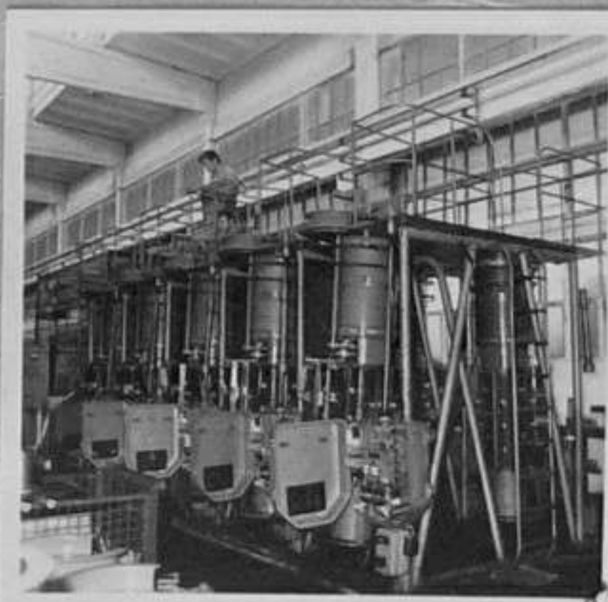
72-4477-12-На стенда за изпитване на стъпалните регулатори РСЗ - 3. /Ан.Цанков/ИК
