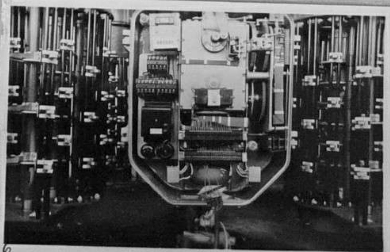
64/3495-3,6 - Нови трансформаторни инсталации, произведени в СТЗ "Васил Коларов" /Ангелов/ ММ
