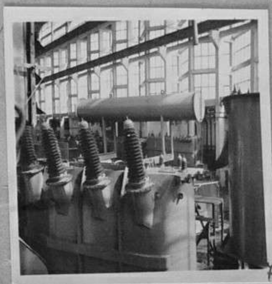
5,7 - Сериенно производство на големи трансформатори.
