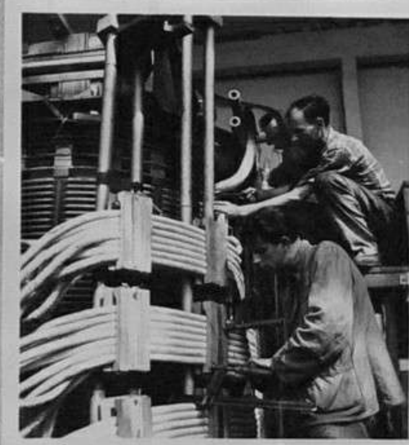
57/2098-1-Монтаж на трансформатор с мощност 31,500 KV. /Халачев/ ММ
