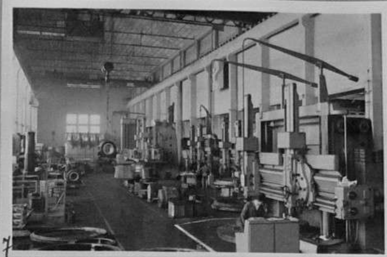
7-Общий вид на генераторный цех в заводе.
