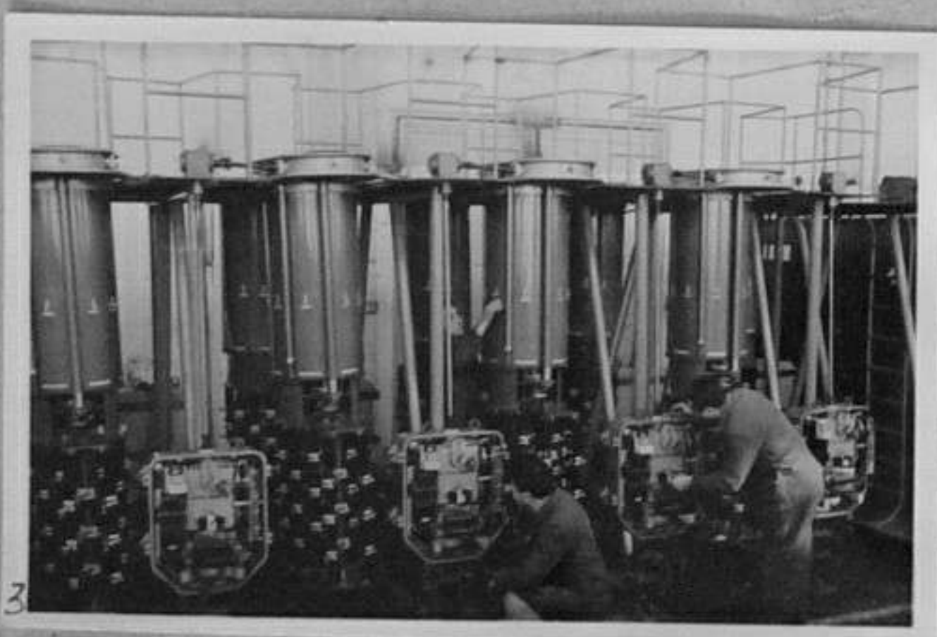
64/3495-3,6 - Нови трансформаторни инсталации, произведени в СТЗ "Васил Коларов" /Ангелов/ ММ
