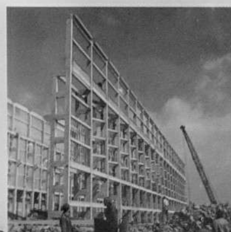
60/2698-2,3 - Строеж на новия трансформаторен цех. /Попов/
