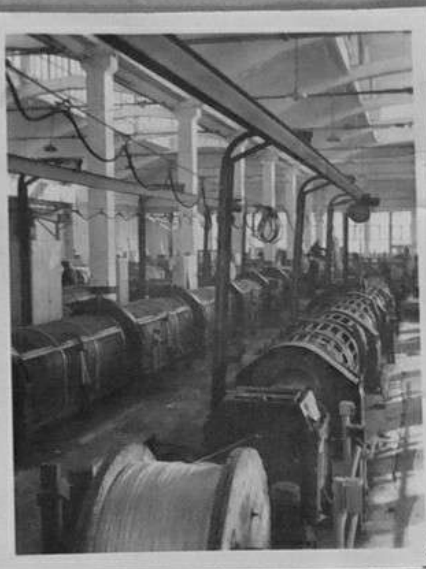
69-60-3-"Торпедо 18"- ма- шина за усукване на жи- ла в цех 300. /Б.Юскеселиев/ XII
