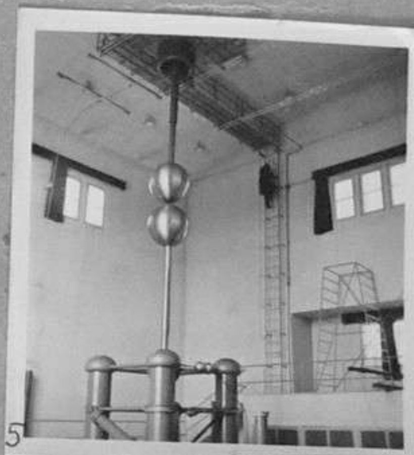
5-Мост за контрола над сферите на височина 16 метра от пода на залата.
