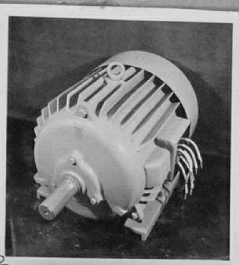
2-Електромотор А02 72-4, дело на инж. А. Пандев и Г. Дончев и конструктор Г. Модев и Р. Ахтимов, има мощност 30 квт, \cos \phi = 0,88 и \eta = 91,5\% . Тежи 245 кг. вместо 310 кг.
