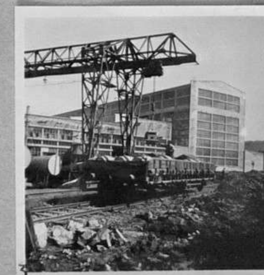
62/677-3- Товарене на вагон с електромотори, произведени в завода. В дъното се вижда новият трансформаторен цех. П. Божков/.
