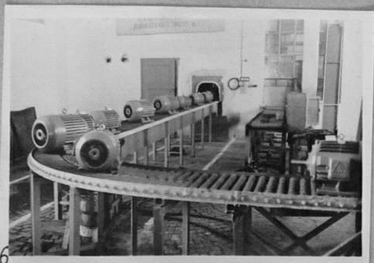
63/3642-6-Пластинчат конвейер за пренасяне двигателите от бояджийския конвейер към ролганга. /Янев/ ММ
