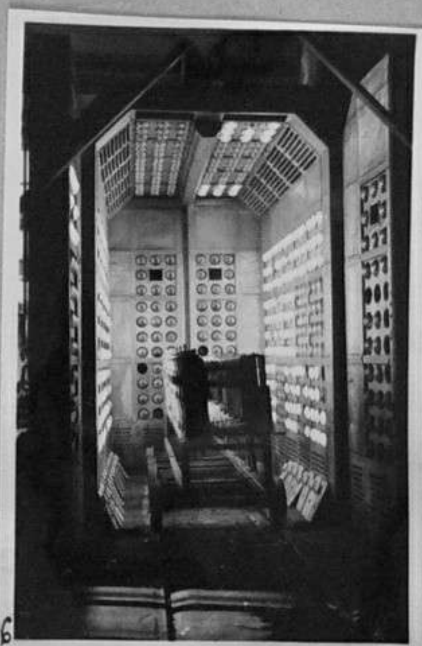
6-Пещ с инфрачервени лъчи за изсушаване на трансформатори и маломаслени прекъсвачи.
