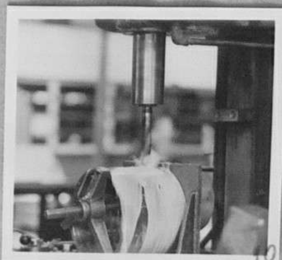
76-2704-10-Автоматична агре- гатна бормашина. /Е.Киров/ЛА
