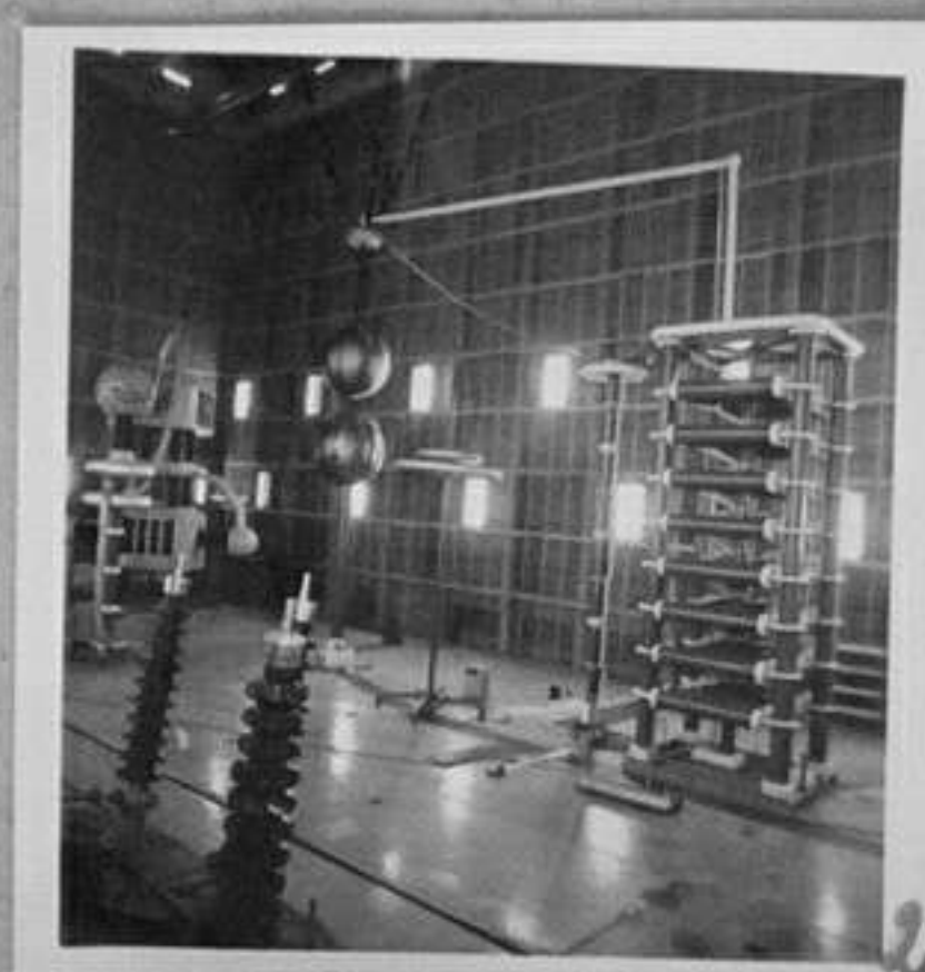
83-1338-2-Изпитателна зала на завод "В. Коларов" и завод "Средец" за изпитване на трансформатори, стъпални регулатори и електрически машини.
