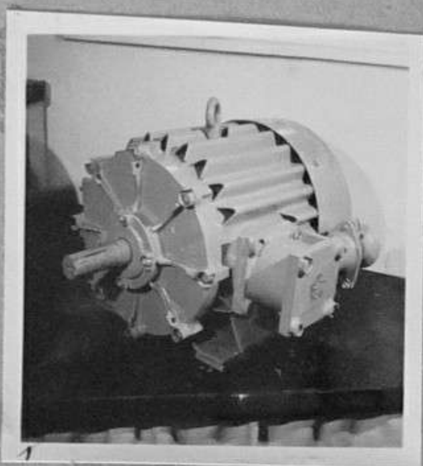
1-Електромотор АВ 71-4, създаден от инж. Вл. Арнаутски и Радомир Радев и конструкторите Г. Зарев и Дим. Ставрев. При мощност 22 квт, \cos \phi = 0,88 и полез. коеф. от 91%, той тежи само 240 кг. срещу 300 кг. при електродвигателите със същата мощност.
