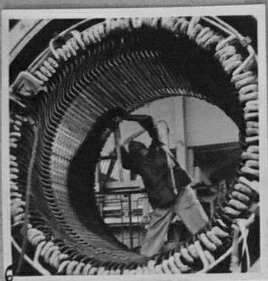
62/2992-6-Изработка на стратор за вертикален генератор с мощност 4250KVA. /Попов/ КМ
