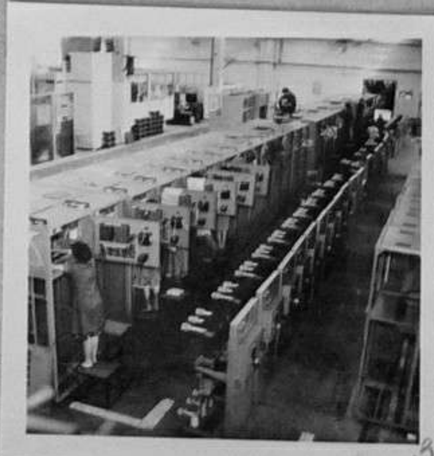
83-1424-2,3-Монтаж на ком- плексно разпределително устройство. В.Балевска/ЛШ
