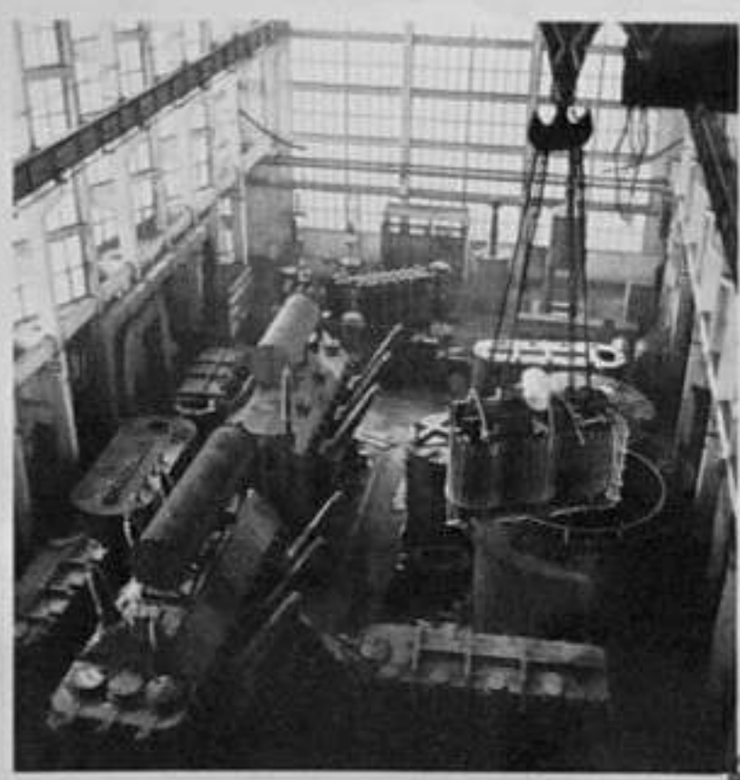
4,5 - Трансформаторно производство. Общи изгледи на цеха за големи мощности.
