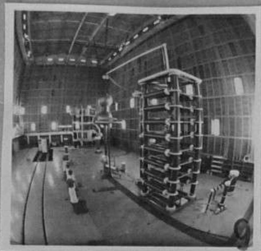
84-63-4, 9, 11-Лаборатория за високоволтово напрежение за изпитание на трансформатори и апаратура на високоволтово напрежение. В. Балева/ЛIII
