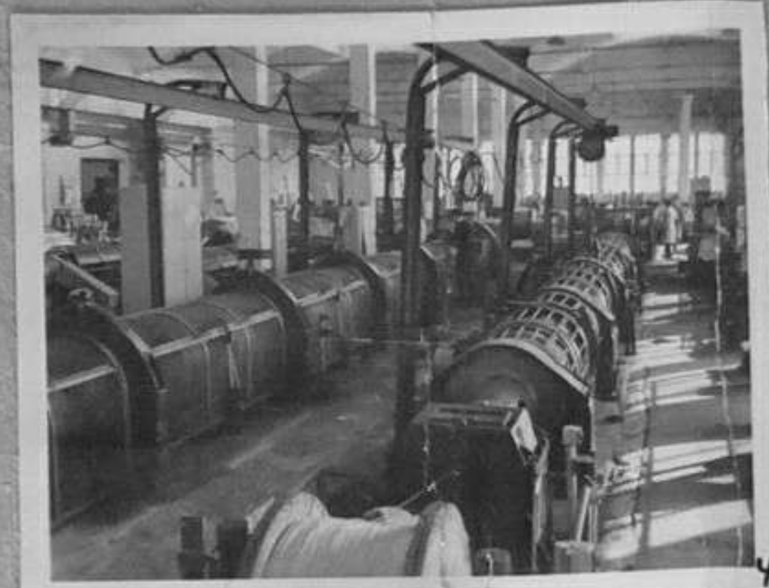
69-60-4 "Торпедо 18" - машина за усукване на жила в цех 300. /Б.Юскеселиев/ XII
