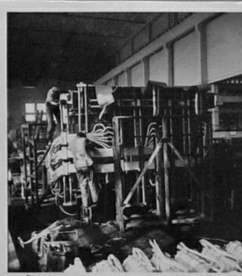
57/2098-1-Монтаж на трансформатор с мощност 31,500 KV. /Халачев/ ММ
