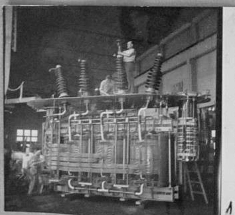
55/1381- 1,2,4 - Новият силов маслен трансформатор 12,500 КВА с двойно регулиране за 110,000 и 20,000 кВ. /Страхинов/
