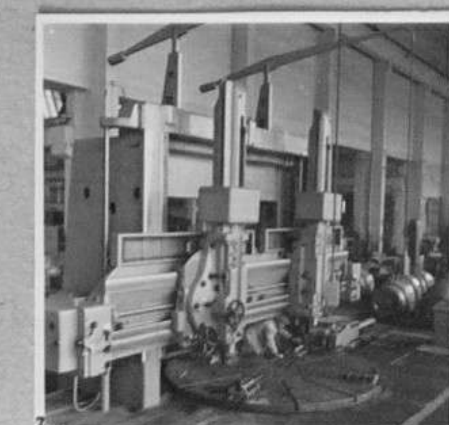
8-Малкият универс.кароселен струг БМН с обща тежест над 110 т.и мощност на двигателя 1100 к.с. е на път за експедиция.
