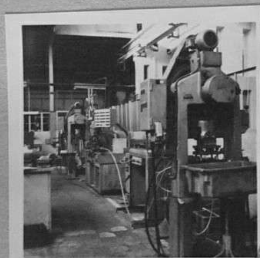
83-1398-4-Поточна линия "Шлатер" за производство на детайли за контакти в цех "Контактни елементи" с началник цех Кузман Василев. Ем. Богоев/ЛШ
