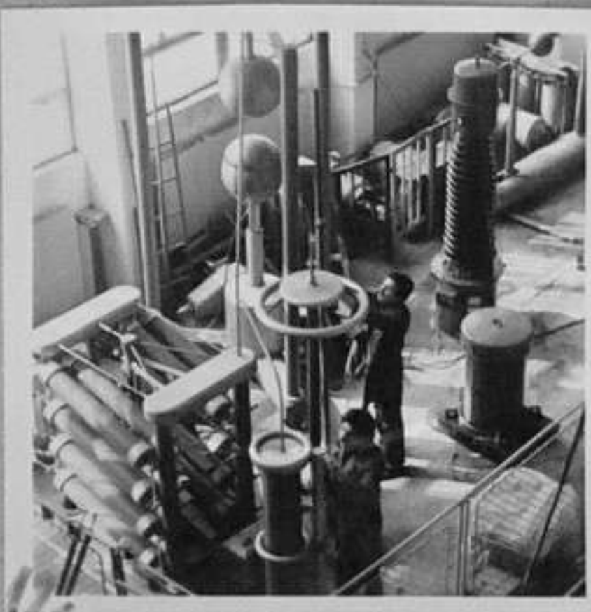
81-516-9,12 Лаборатория за изпитване на трансформатори, предназначени за износ и вътрешния пазар
