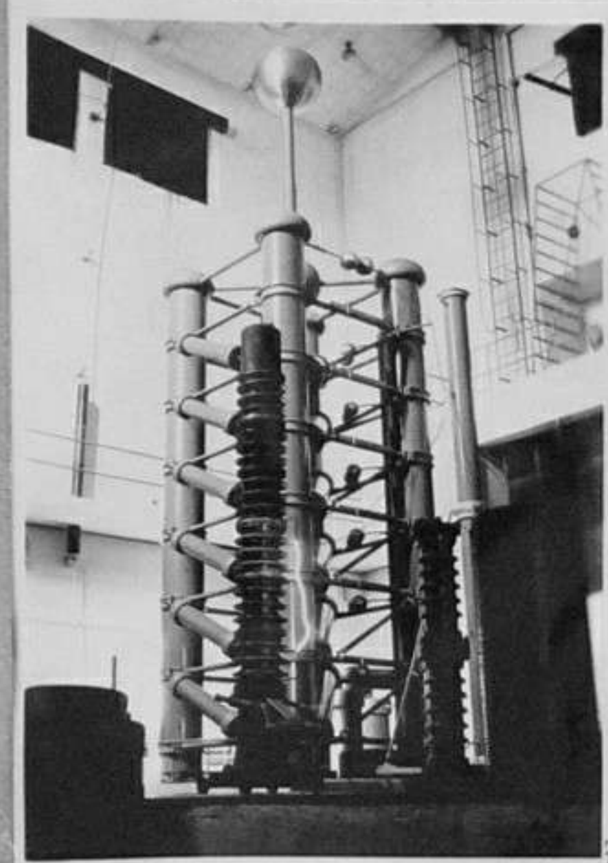
59/324-4-Изпитания на високоволтови апаратури под напрежение от 100,000 до 1200000 волта. /Страхинов/
