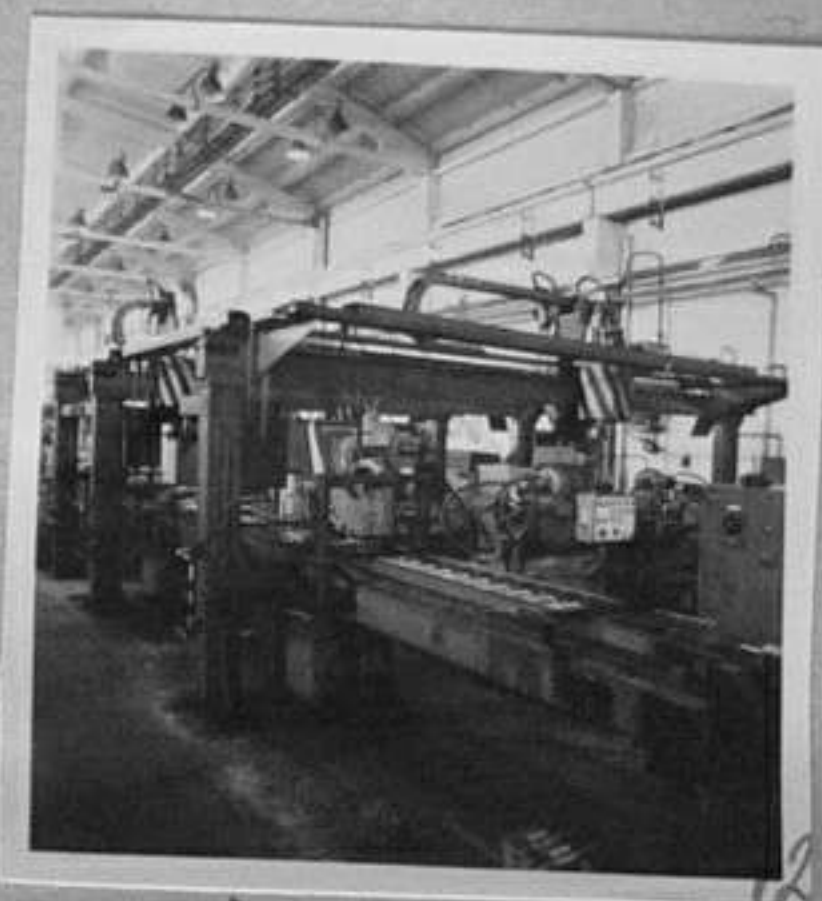
83-762-12 Автоматична линия за обработка на вал с ротор Е. Любомиров/МД
