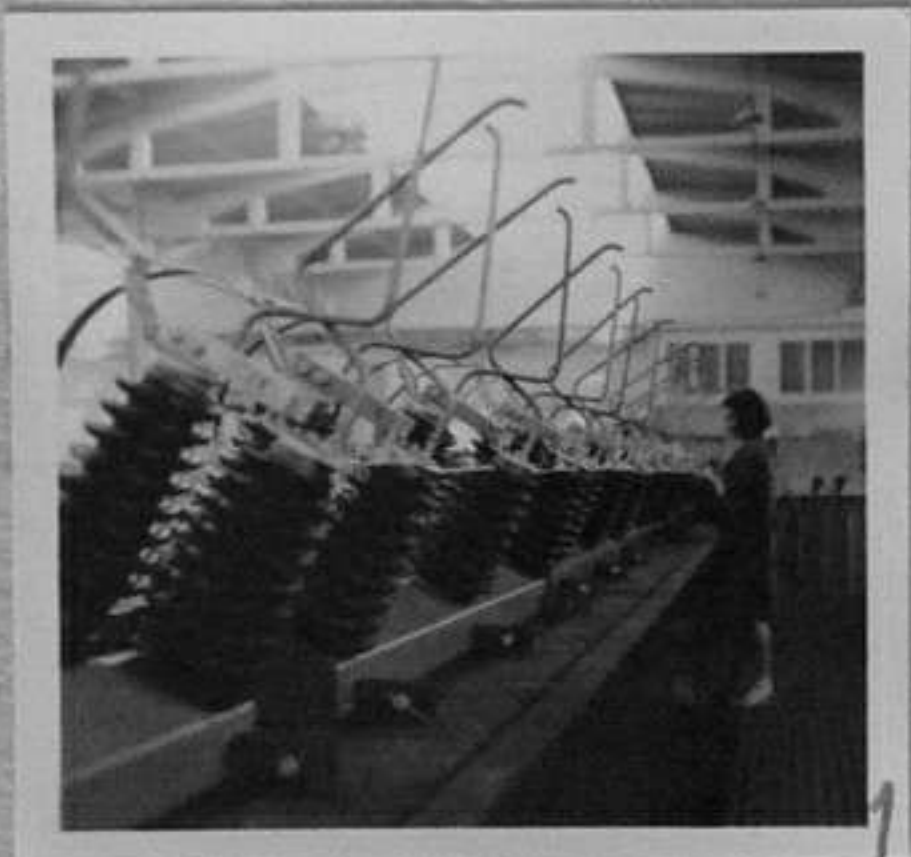
73-3383-1, 4, 6-Монтаж на секционен разединител тип "Рос" 20/200. /Д.Рогов/ТК
