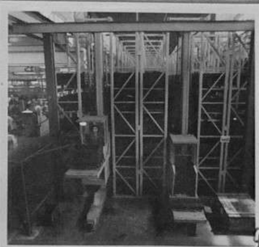
73-1467-9-Предмонтажен палетизиран склад, съоръжен с трансманипулатори. /АН.Цанков/ЕИ
