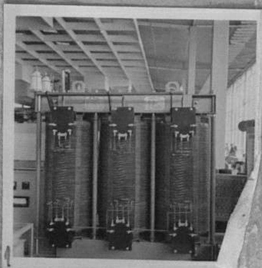
67-3361- Щандът на Н И П 1- Сух трансформатор тип ТС 400/10 за вграждане в трансформатор на подстанция.
