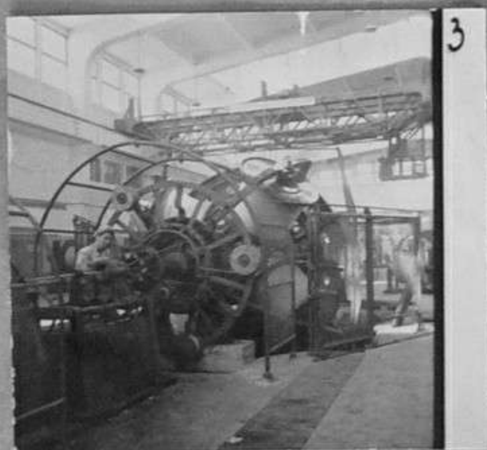
2-3 - Кабелният цех - производство на армиран кабел. 5-Панцeroва машина.
