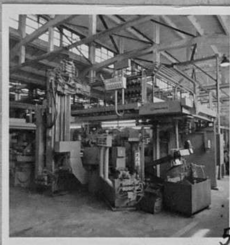
77-2367-5- Автоматична по- точна линия за обработка на лагерен щифт. /В.Балевска/ЛА
