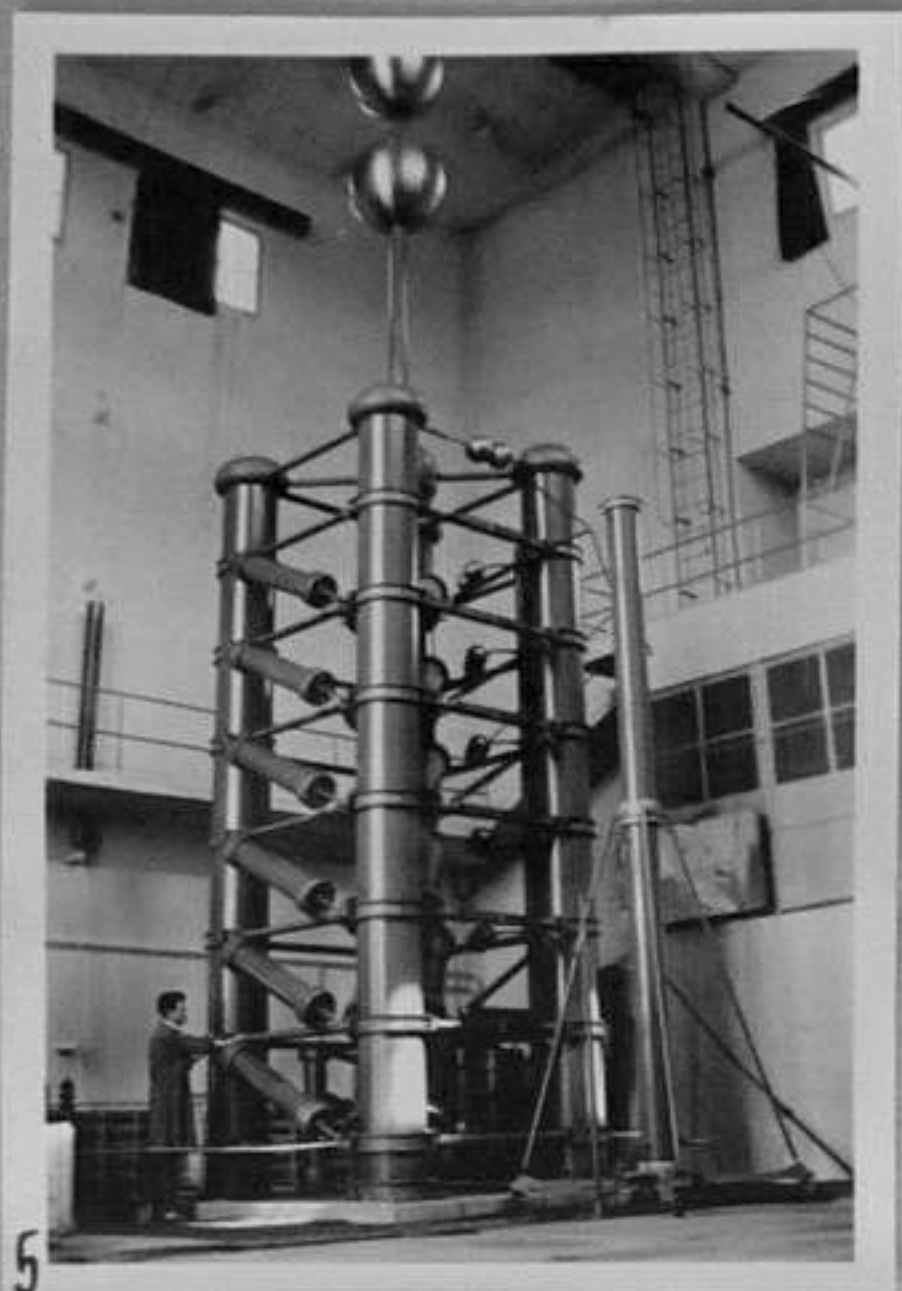
5-Импульсный генератор мотор ВМ.
