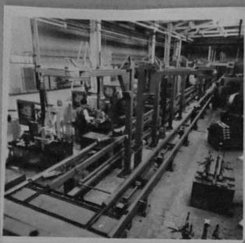
83-1339-5-Автоматизирана линия за механична обработка на ротори за електродвигатели. Р. Марукян/ЛШ
