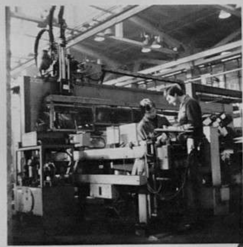
80-3489-2,7 Участък "Валове" - автоматична линия за шлайфане на валове с оператори-настройчици Лъчезар Велинов и Владимир Христов Кр.Узунова/МД
