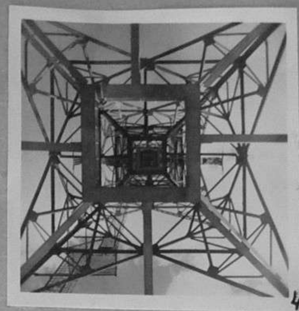
68-4683-2,3,4-Електрически стълб от далекопровода Румъния-България. /И.Хаджимишев/ XII
