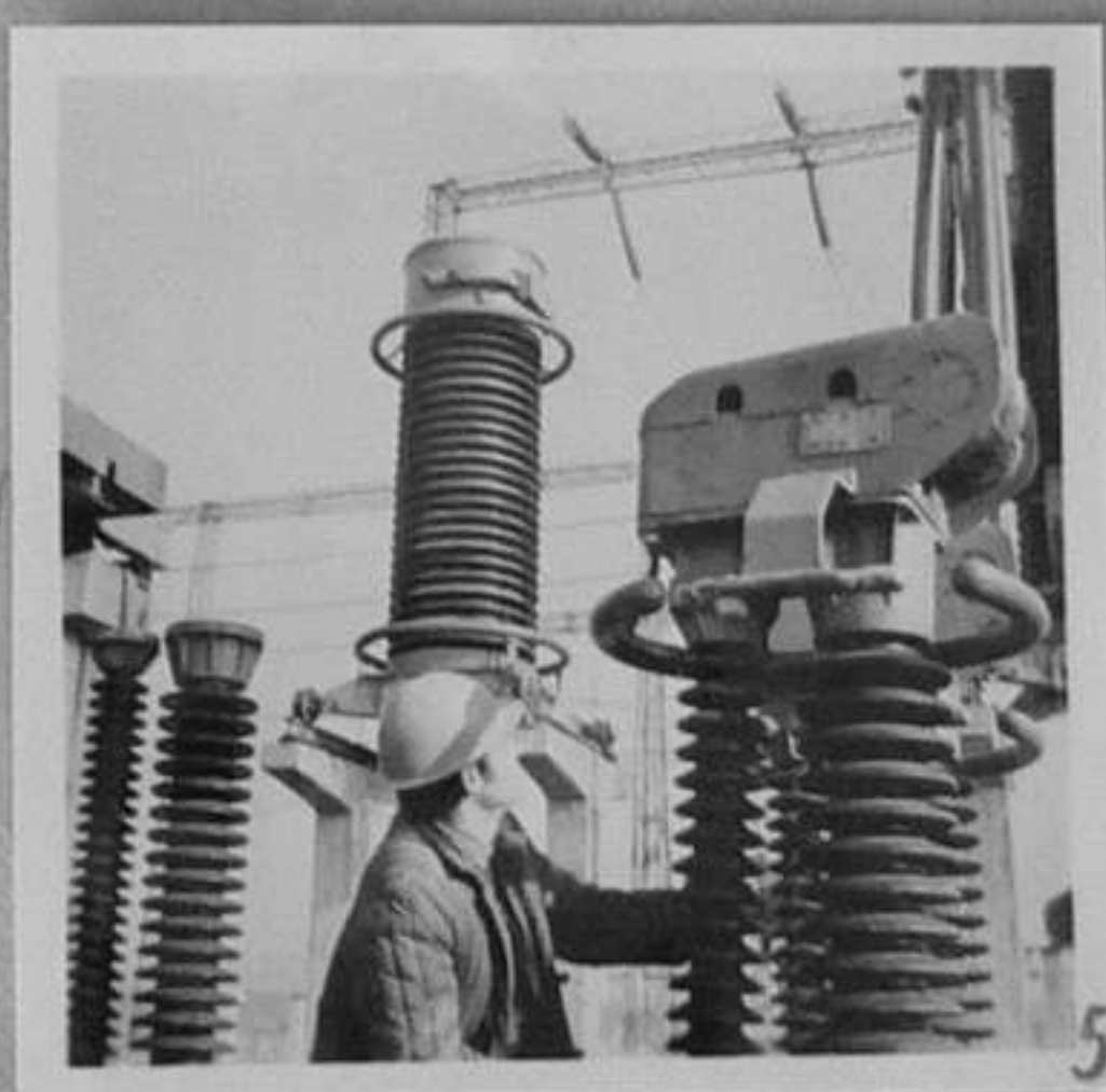
71-669-1,4,5-Монтиране на ножови разпределители на подстанцията "Мизия" към далекопровода "Дружба". /Л.Златков/ ХП
