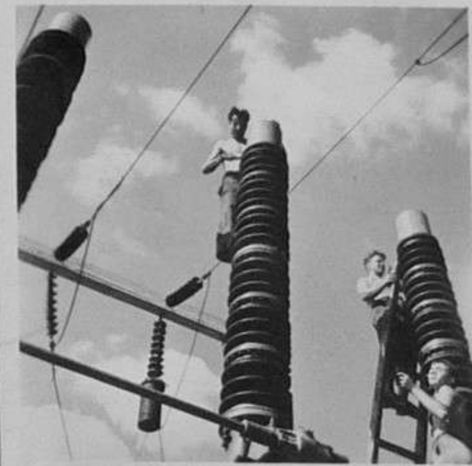
57/2281-9,11 - Монтаж на маломаслени прекъсвачи 110 кВ на подстанция Горна Оряховица, която се свързва с далекопровода "Алеко Константинов". /Хорисан/
