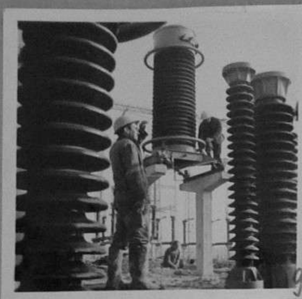
71-669-9-Монтиране на ножови разпределители на подстанцията "Мизия" към далекопровода "Дружба". /Л.Златков/ ХП
