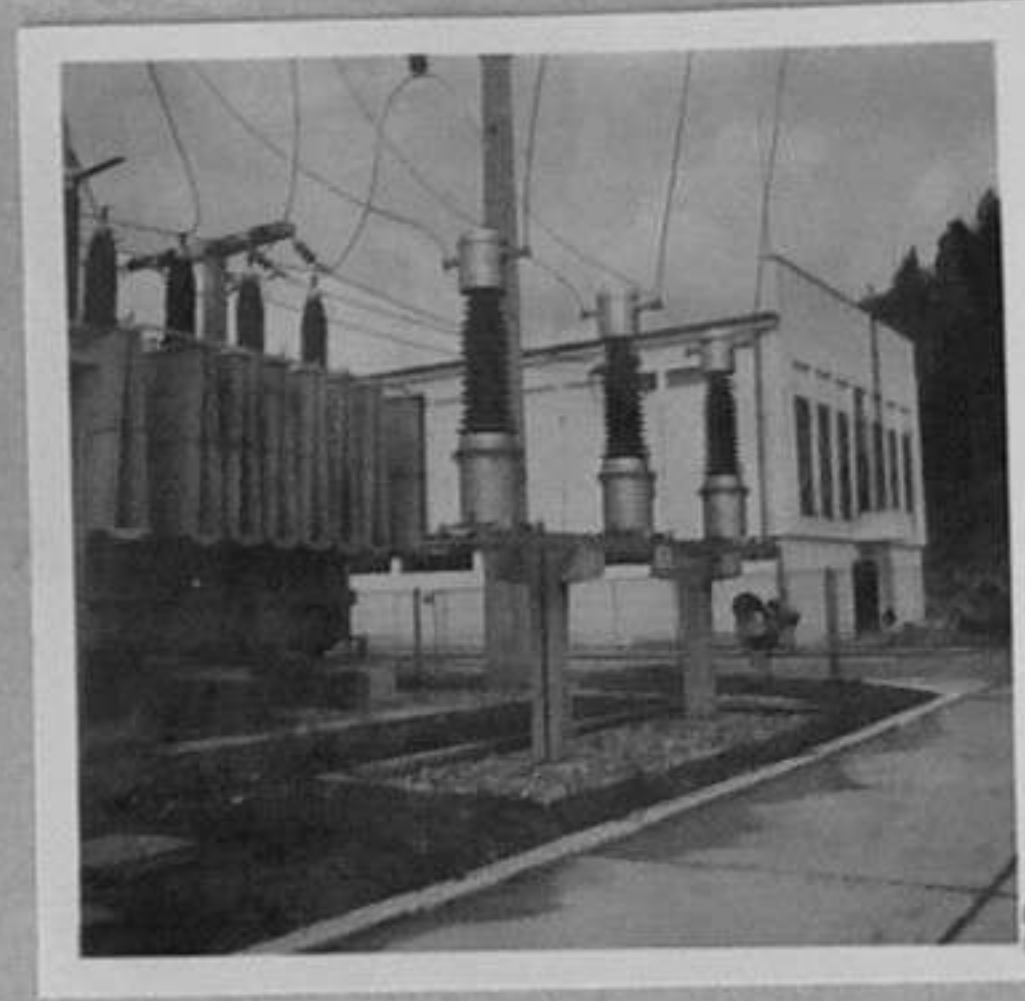
72-4204-8-Общ план на под- станция Котел,открытата уред- ба и трансформатора. /Е.Богоев/МК
