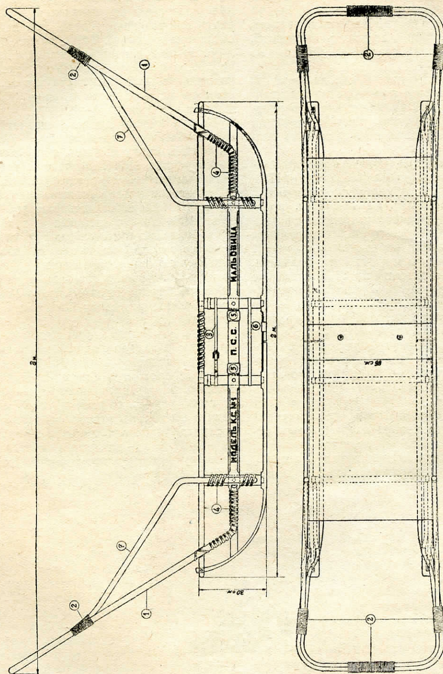
Конструкция на новия моделъ спасителна шейна
