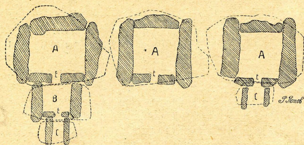
2. Планове на три типа долмени А. Камара. В. Предкамара. С. Коридор. Е. Входи.
